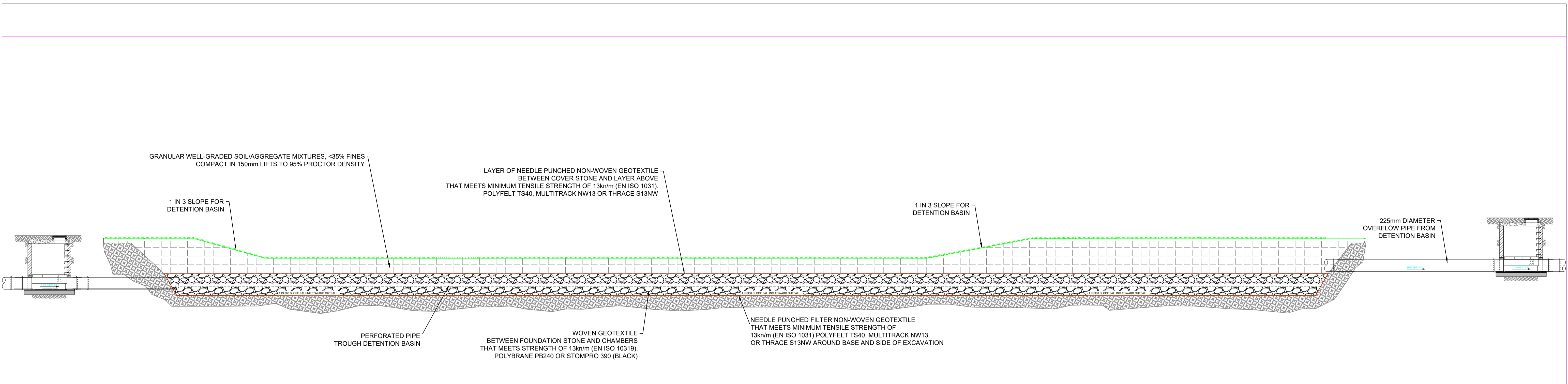
DETENTION BASIN SECTION A-A SCALE: 1:60
