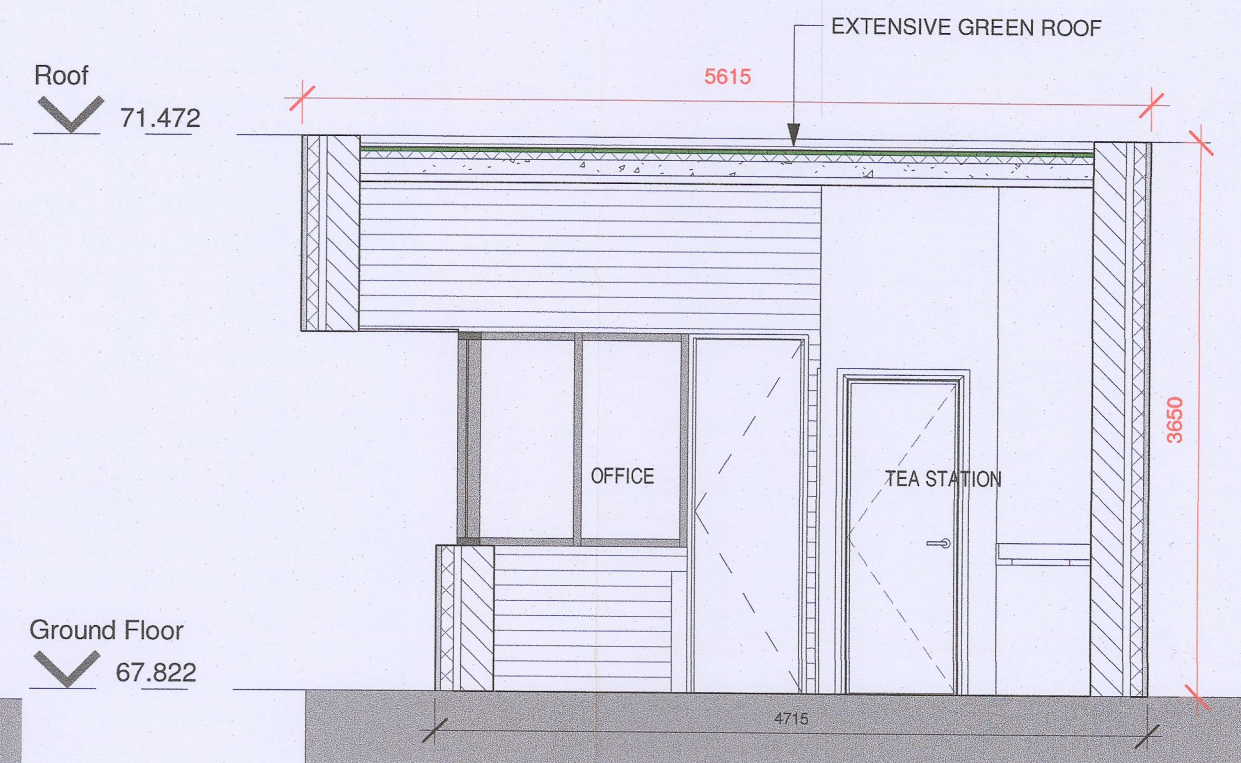
4 6523 Section 2 1:50
