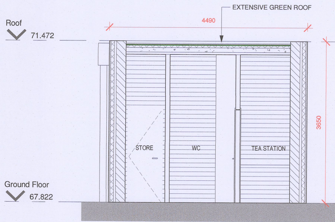
3 6523 Section 1 1:50
