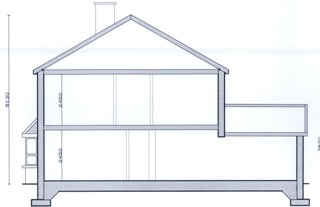
EXISTING SECTION A-A SCALE 1:100 @A3
