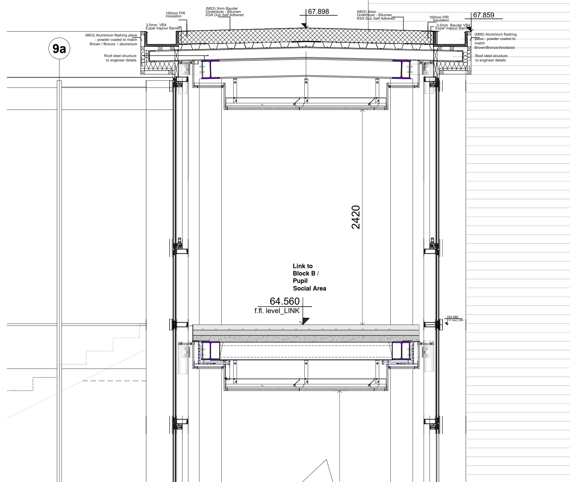
KEY ELEVATION - DET 1 - 1:25
