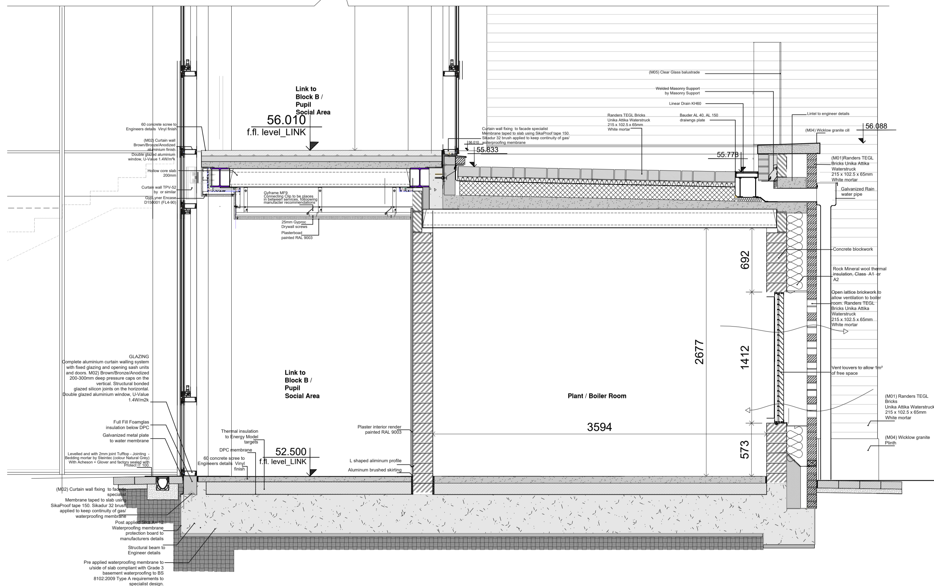
KEY ELEVATION - DET 2 - 1:25
