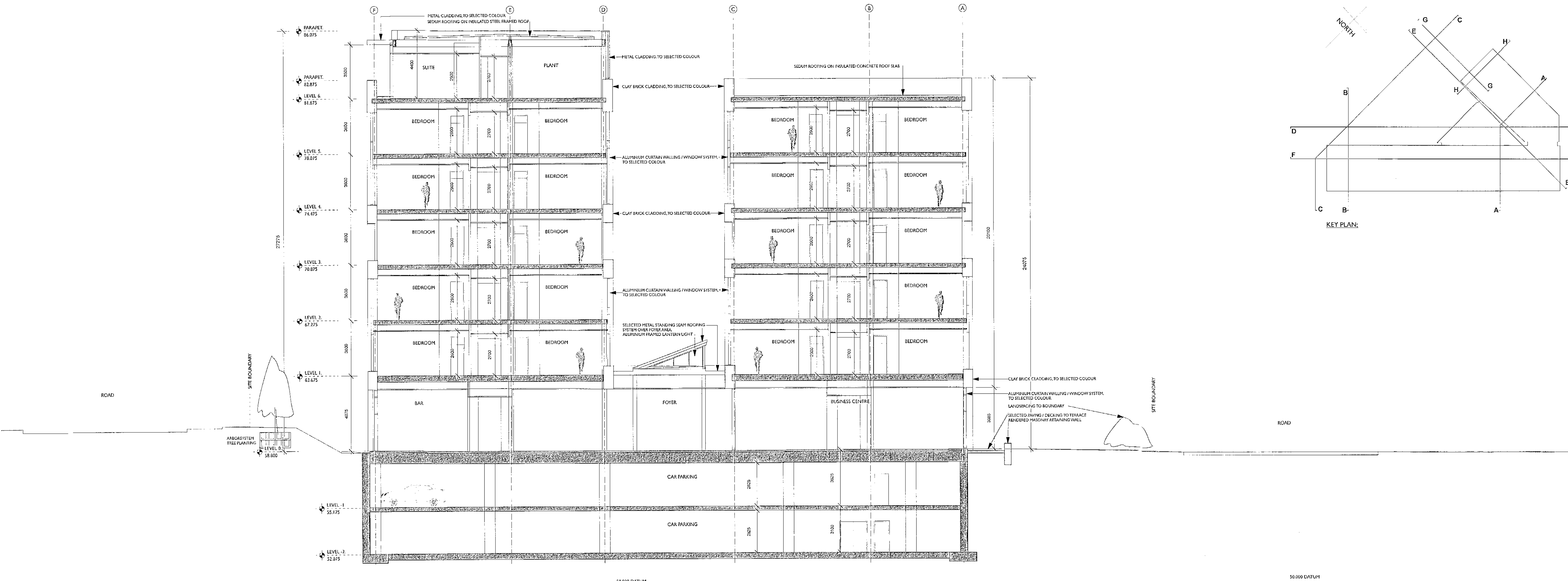
SECTION A-A
