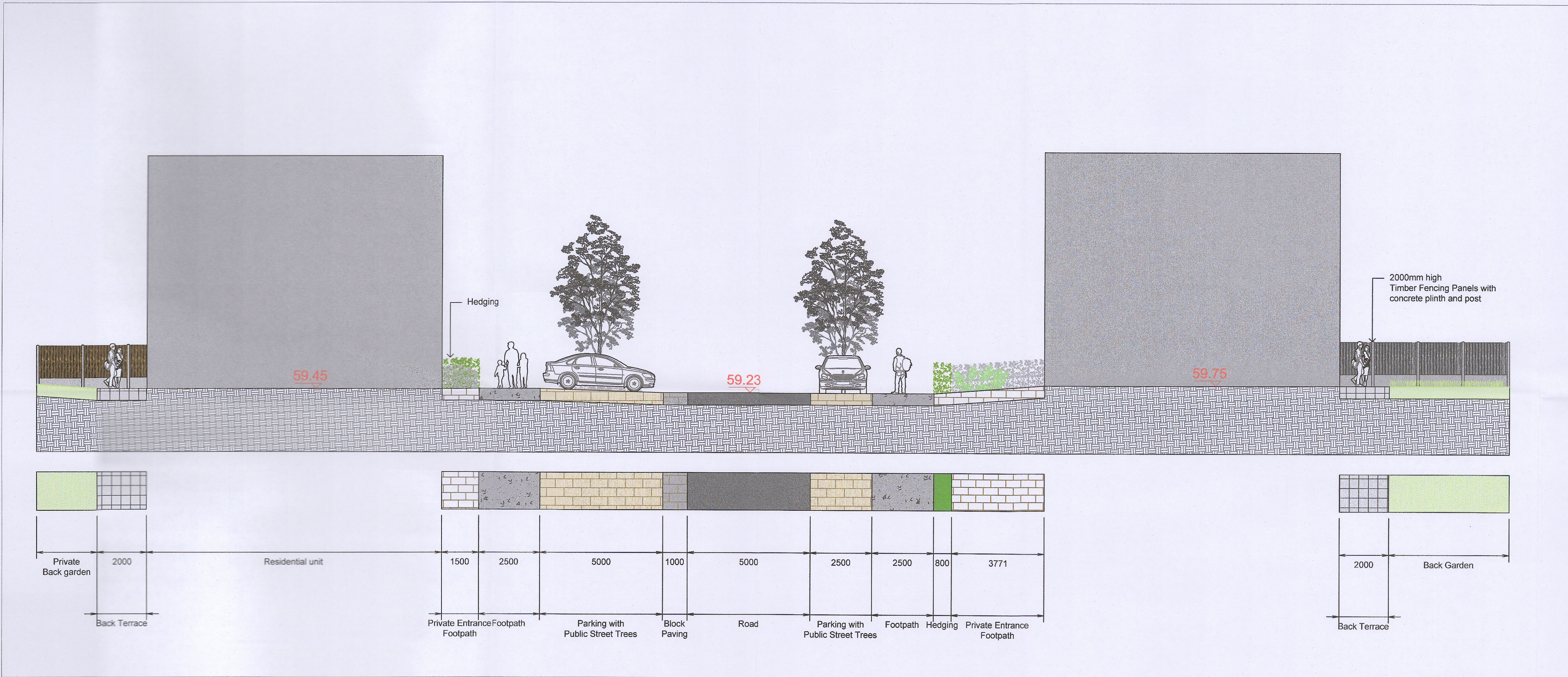
C Section SCALE: 1:100 @ A1
