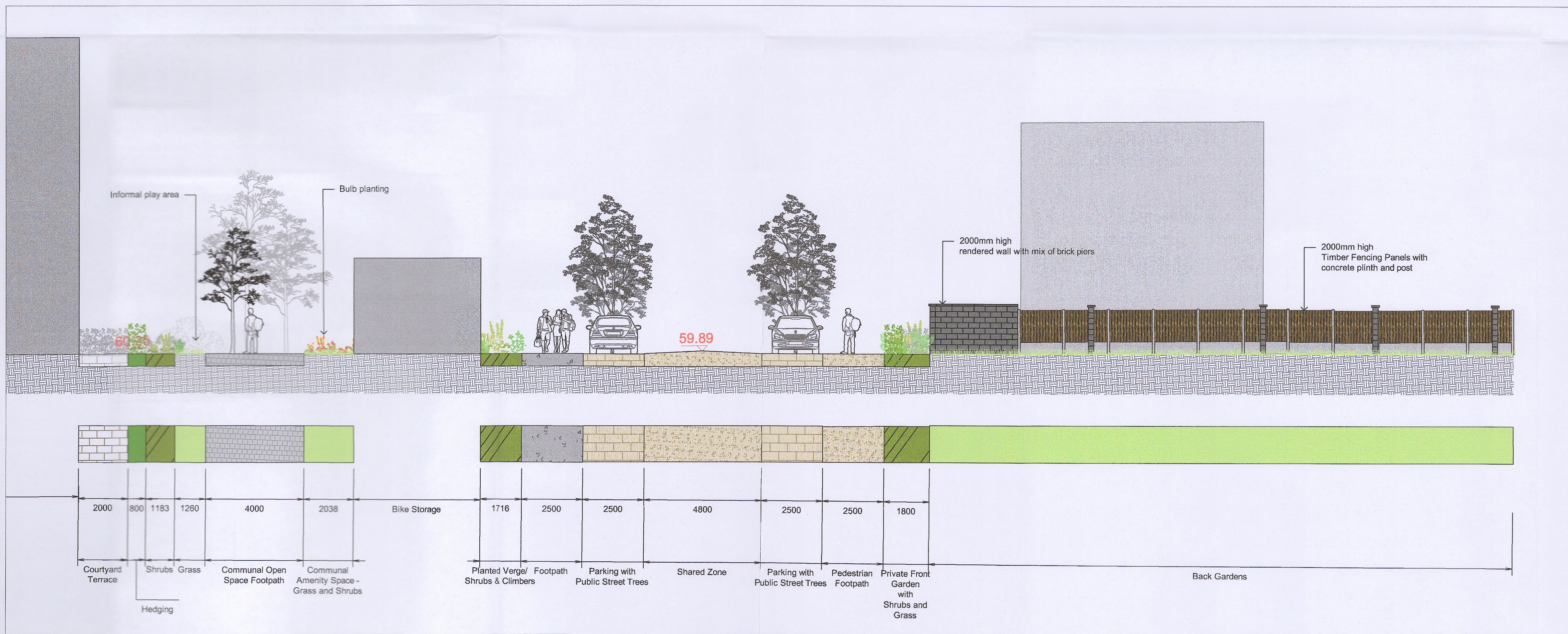
A Section SCALE: 1:100 © A1
