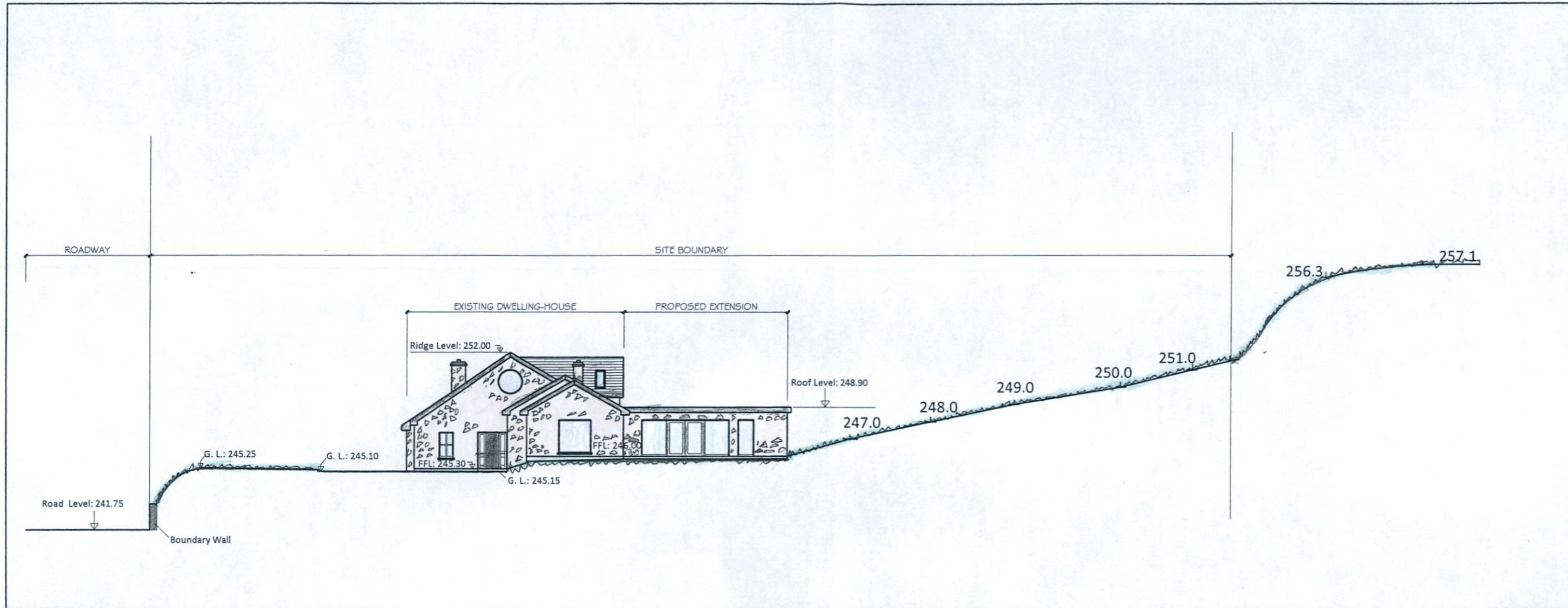
SITE SECTION A-A SCALE 1:250 (A3)
