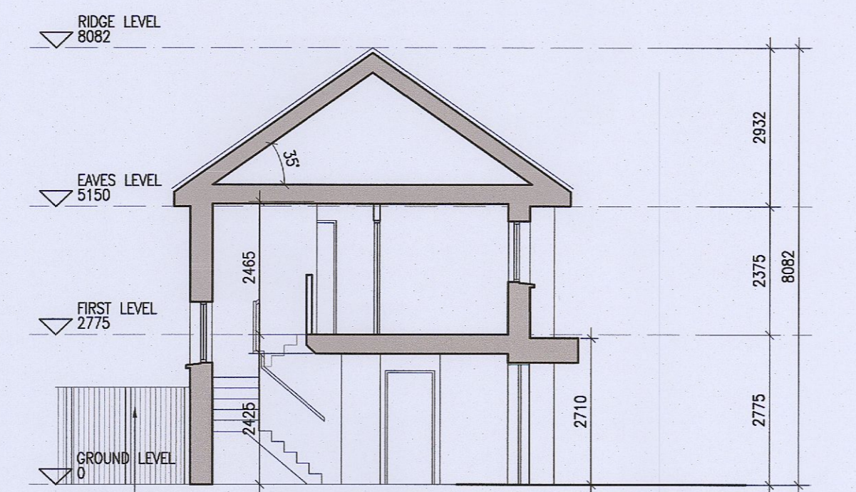
07 Section A-A
