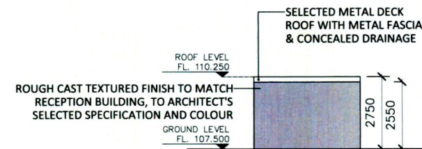
02 ELEVATION 01 PA500 1:200
