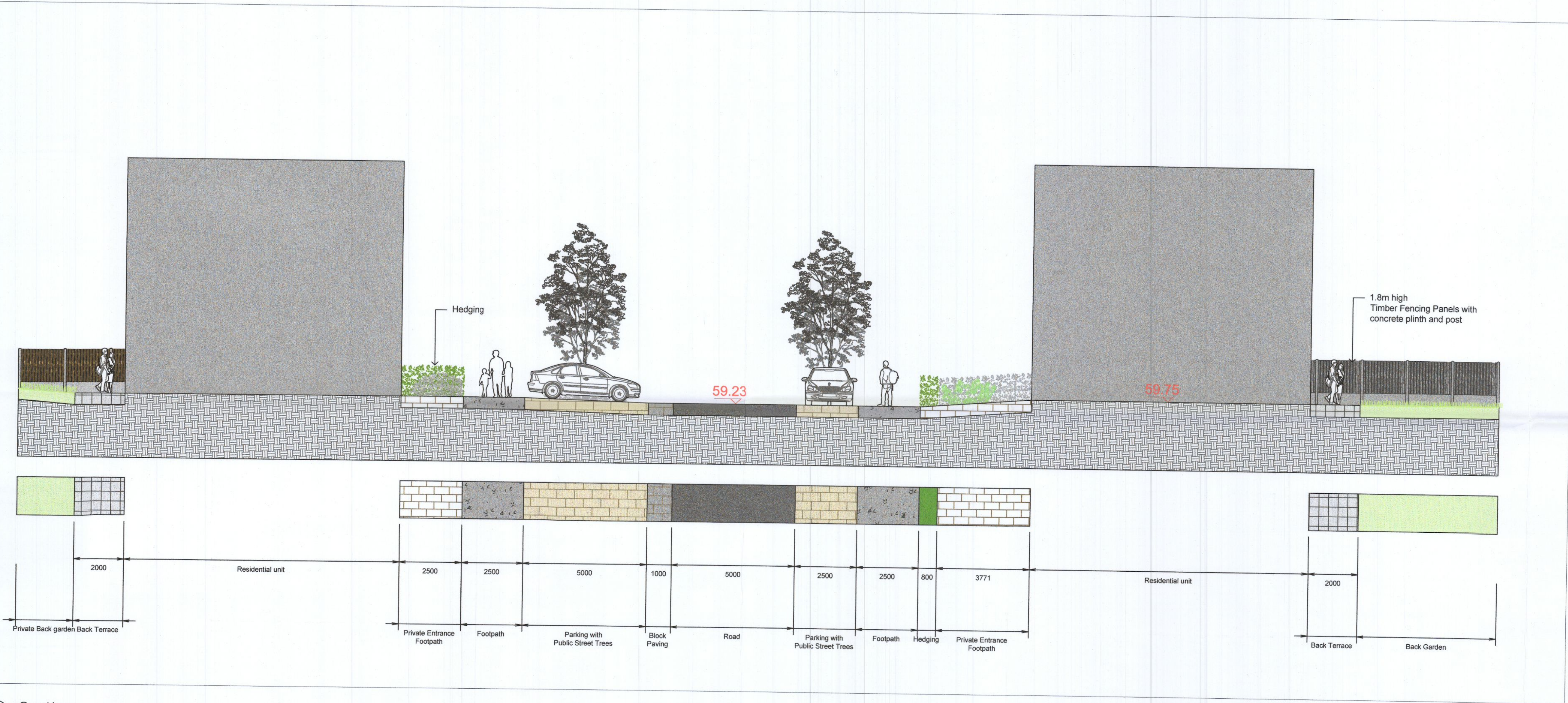
C Section SCALE: 1:100 @ A1
