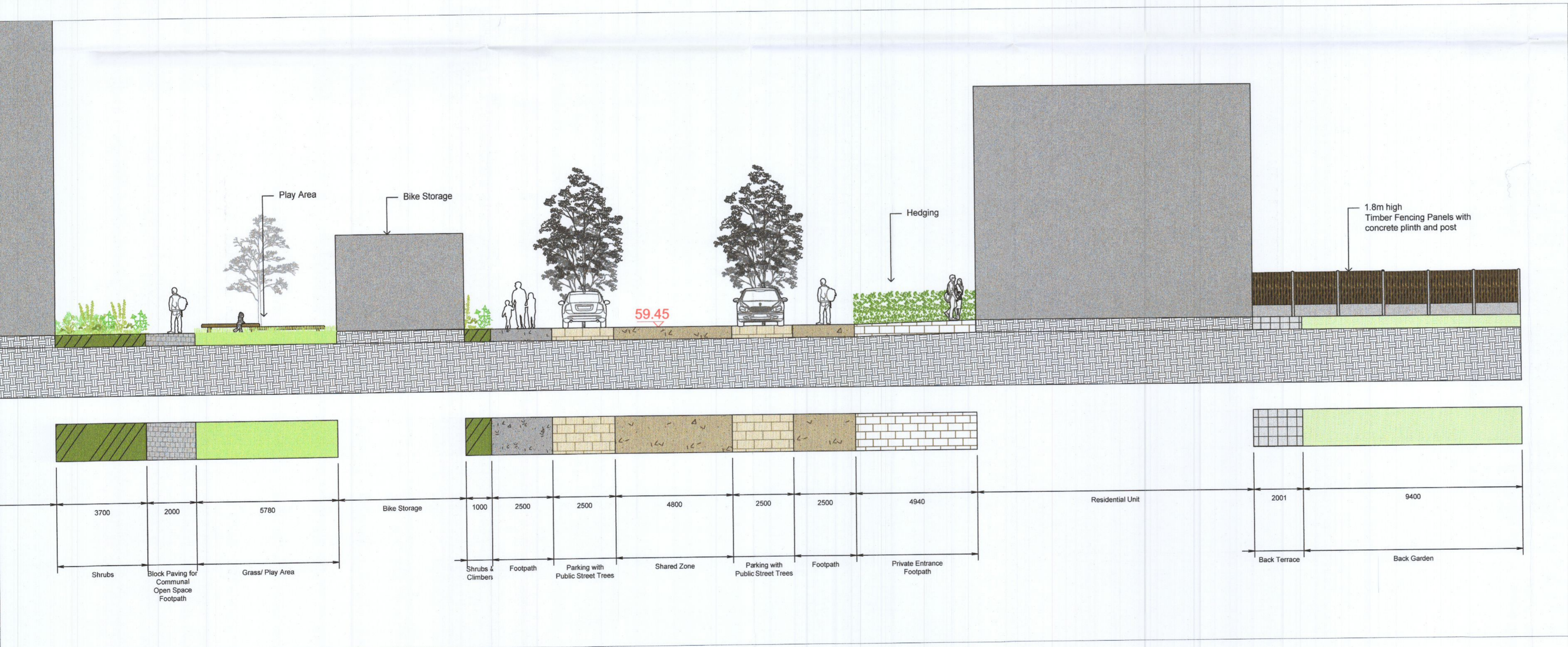
B Section SCALE: 1:100 @ A1
