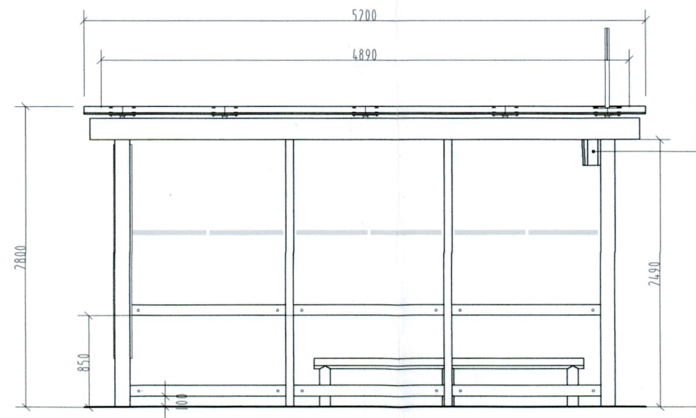
RERE ELEVATION
