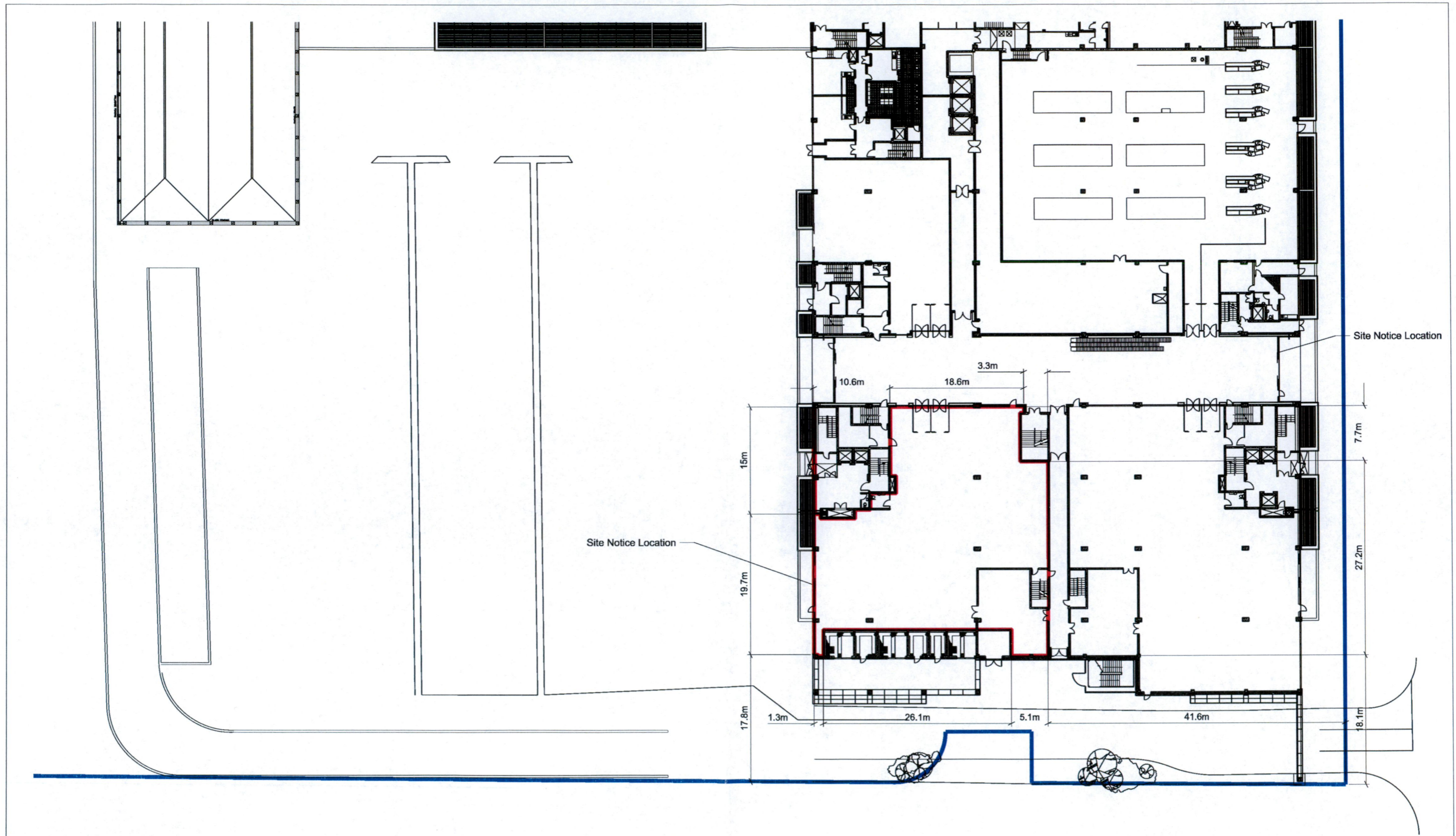
1 SITE PLAN 1:200
