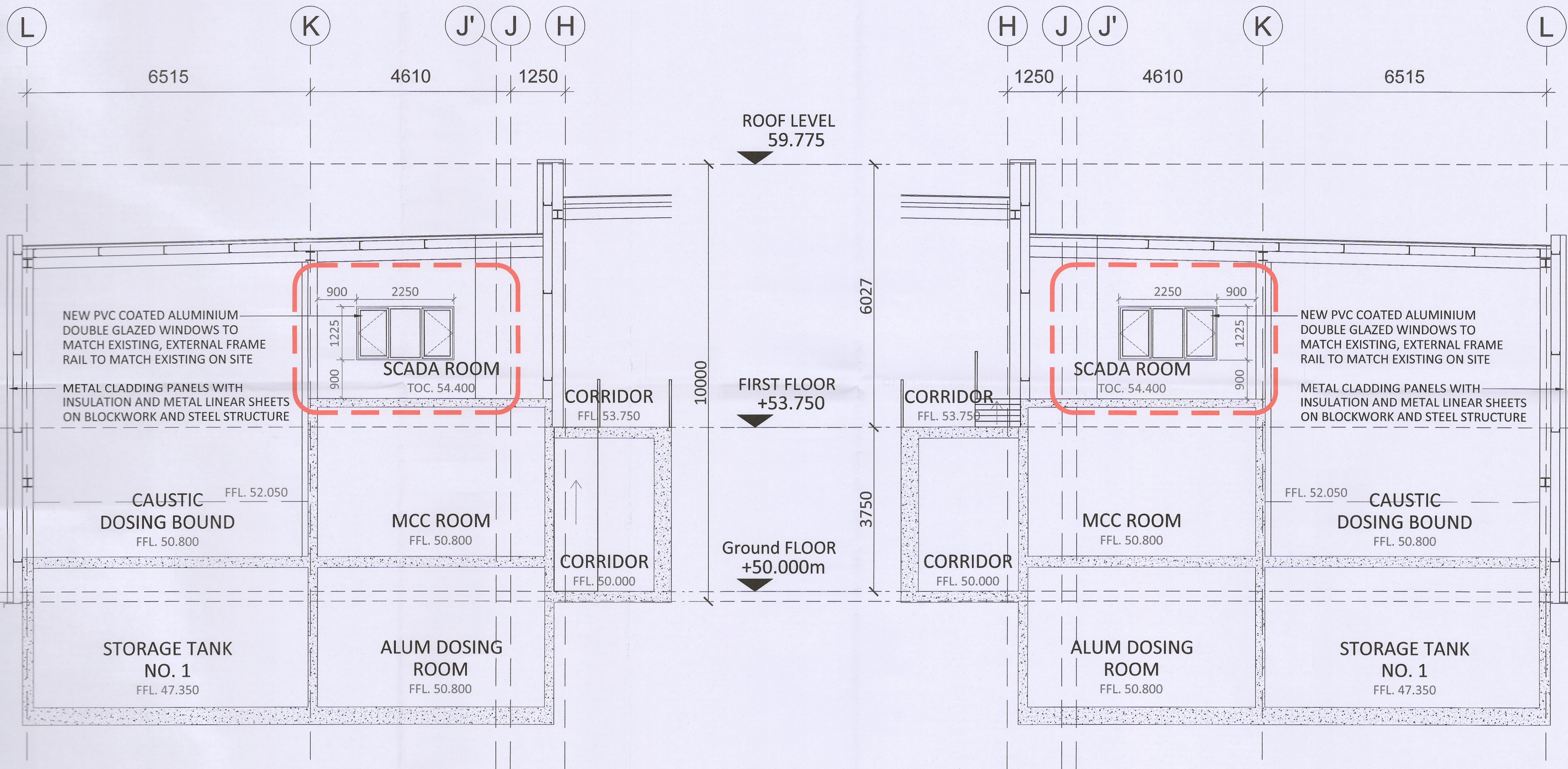
01 SECTION 1-1 SCALE: 1:50@A1
