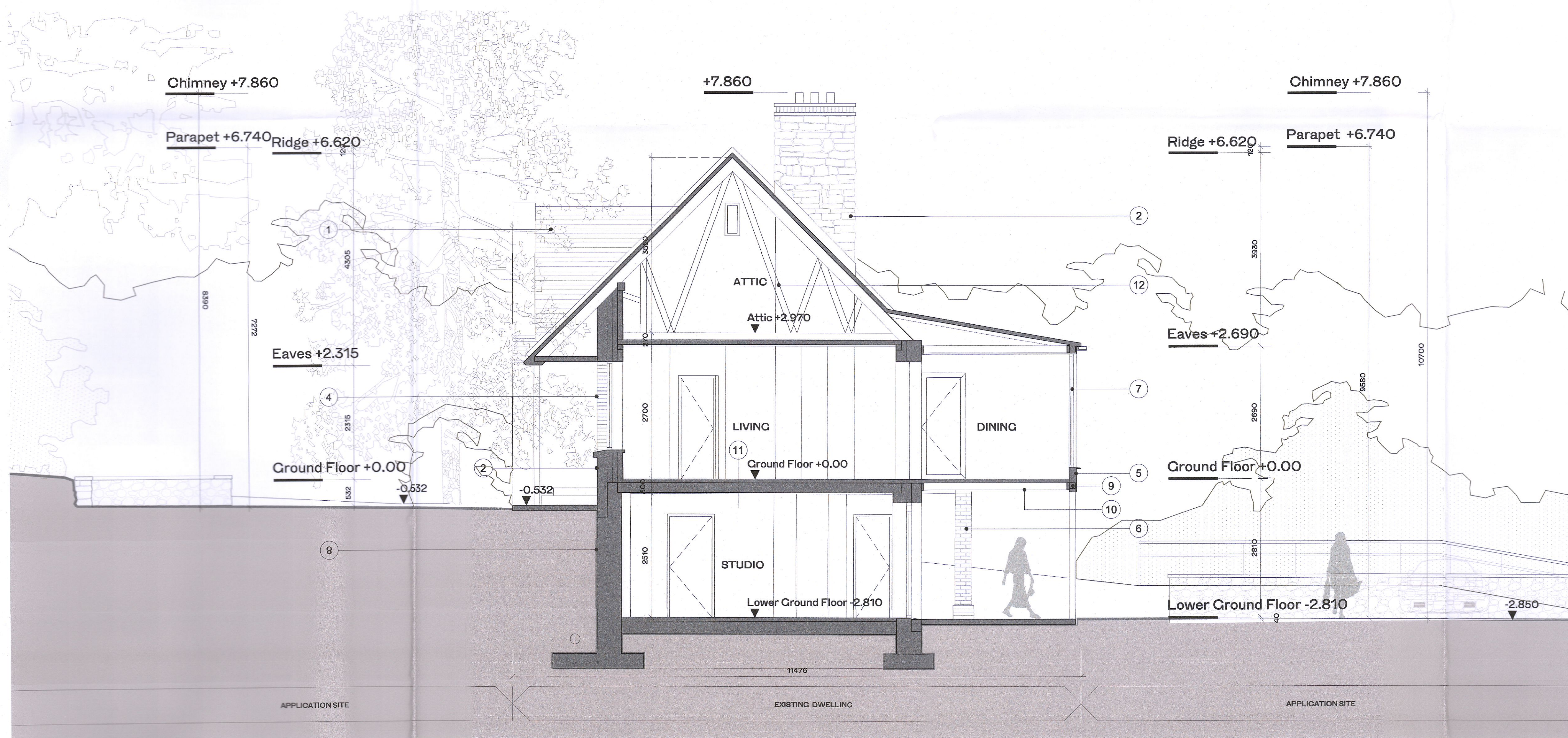
SECTION A-A - EXISTING - 1:50
