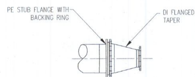
PE TO DI DETAIL SCALE 1:20
