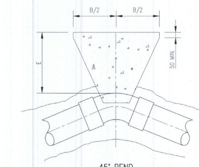
45° BEND
