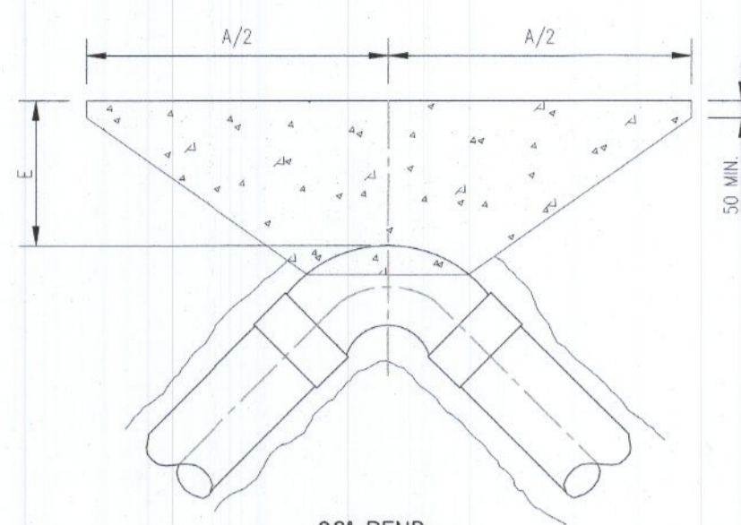
90° BEND
