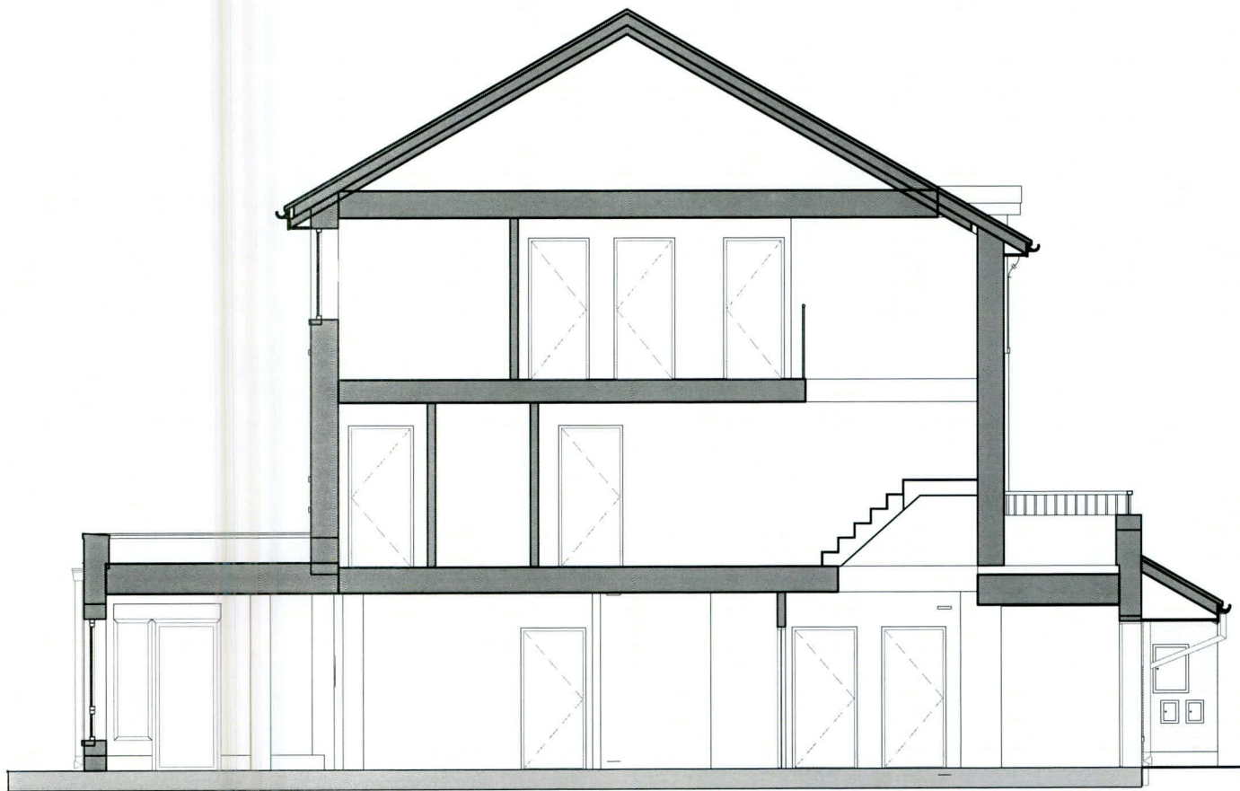
1 Unit Type D Section AA 1 : 100
