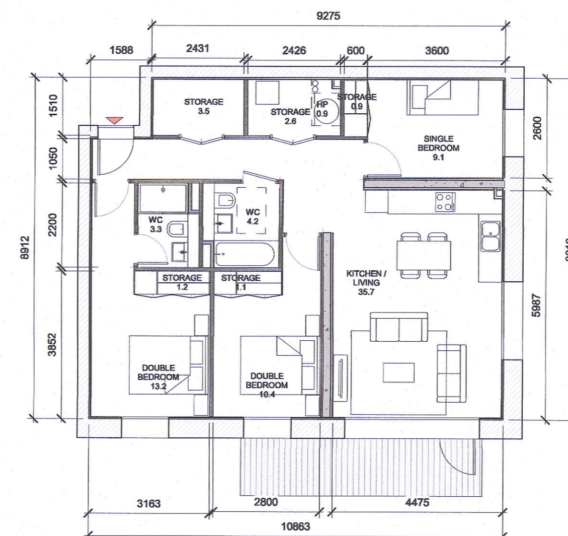
3 T.301_C 1:100
