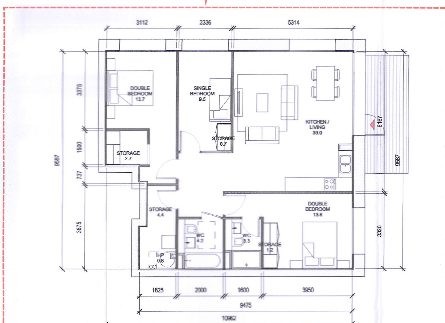
4 T.301_D 1:100
