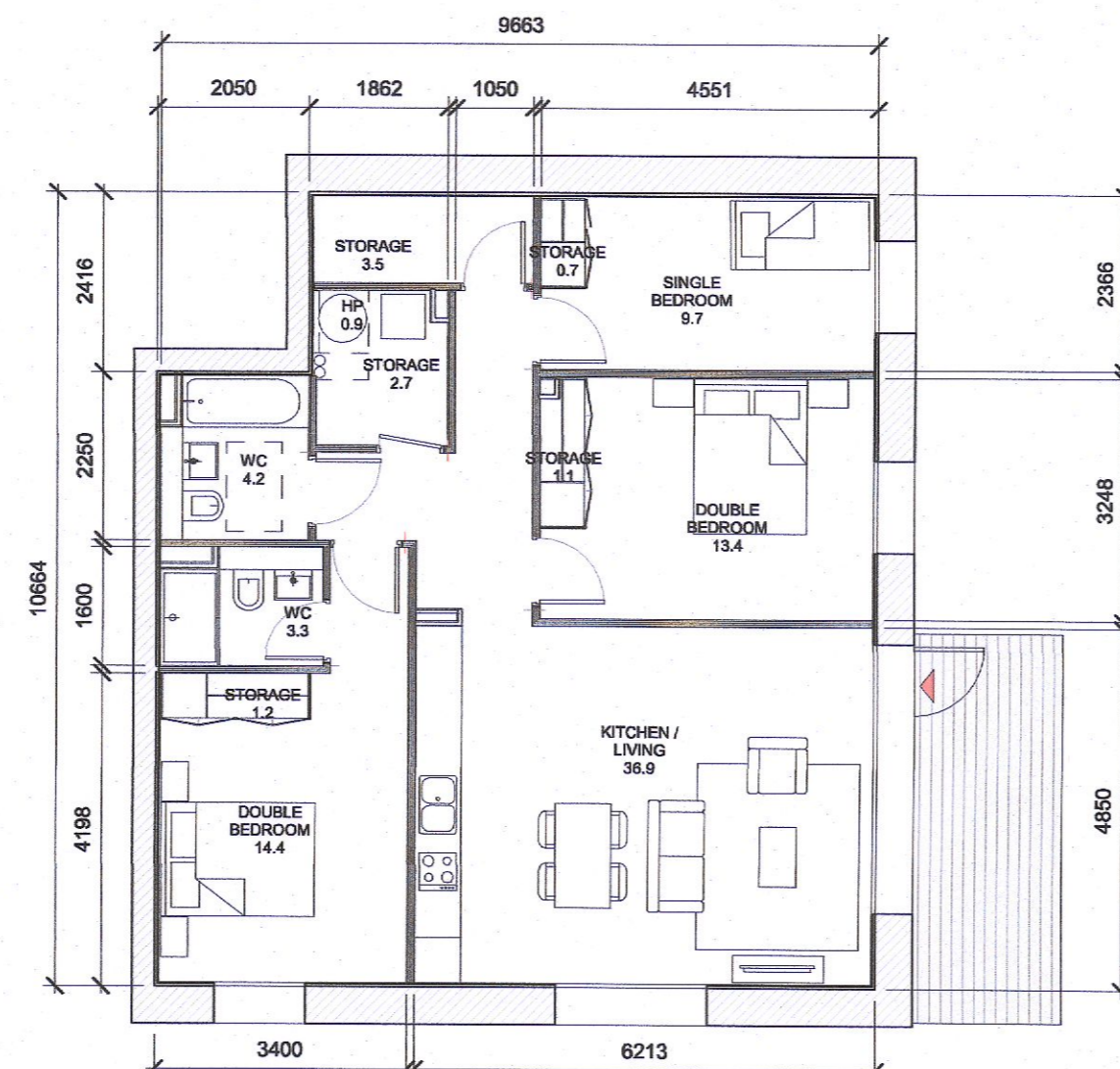
2 T.302_A 1:100
