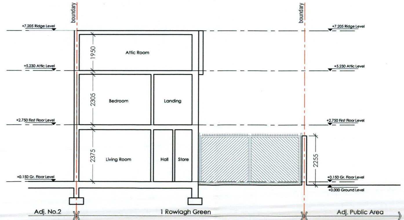
003 Section A-A - EXISTING 04 1:100
