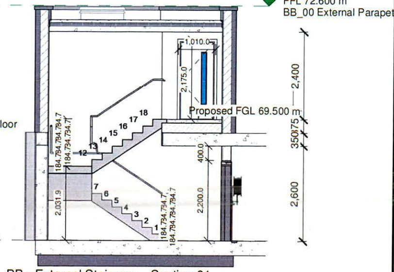
BB - External Staircore _ Section 01 1 : 100
