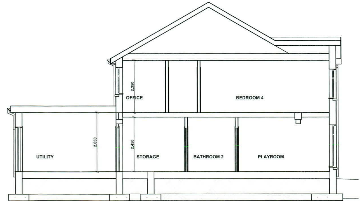
Section D-D 1:100
