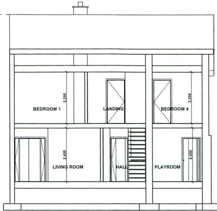
Section A-A 1:100
