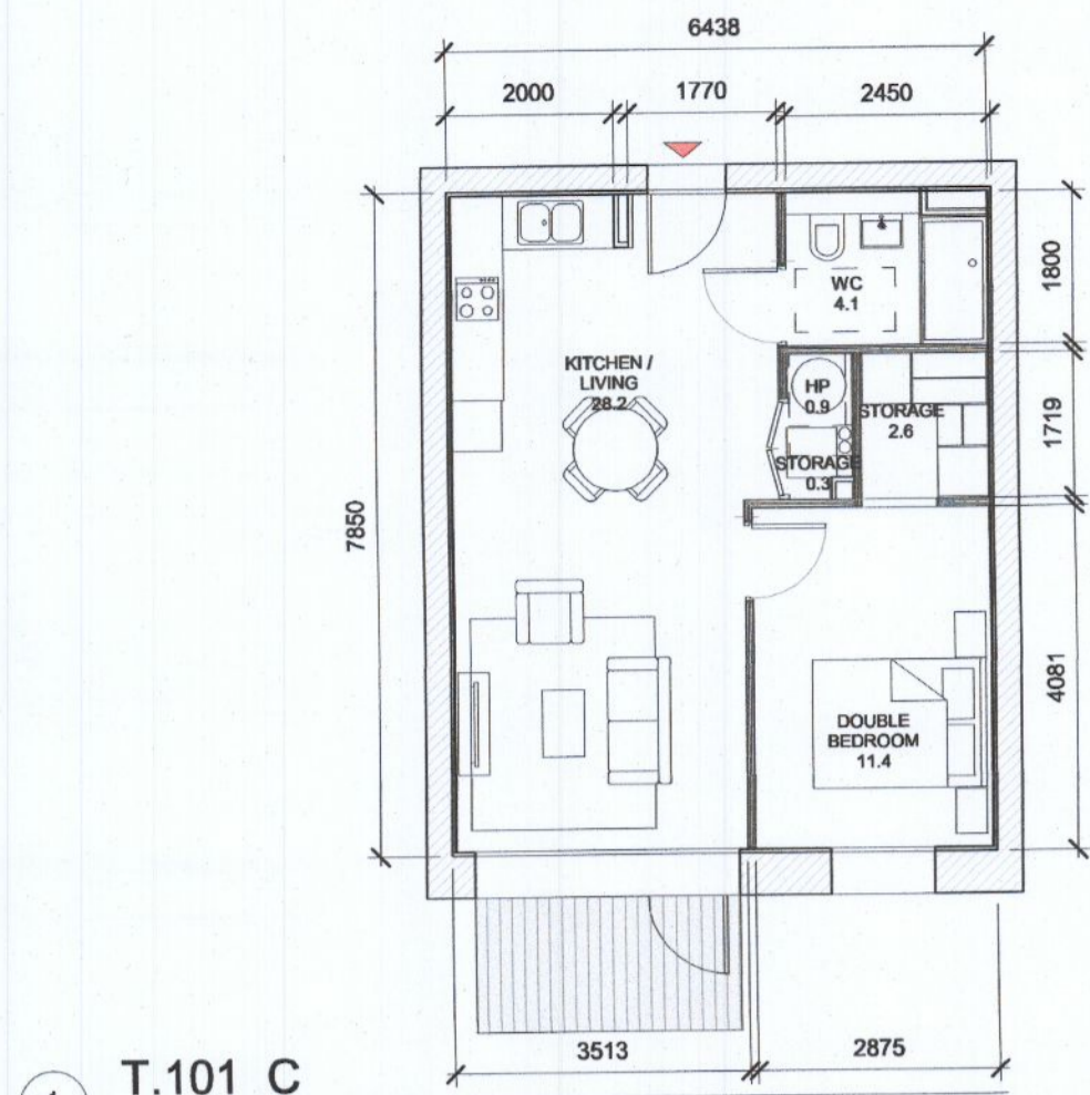
1 T.101 C 1:100
