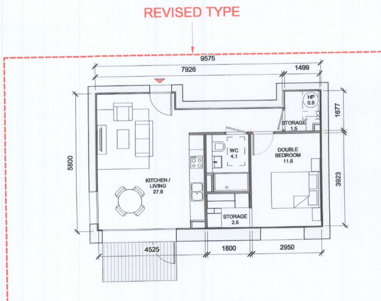
10 T.102 D 1:100
