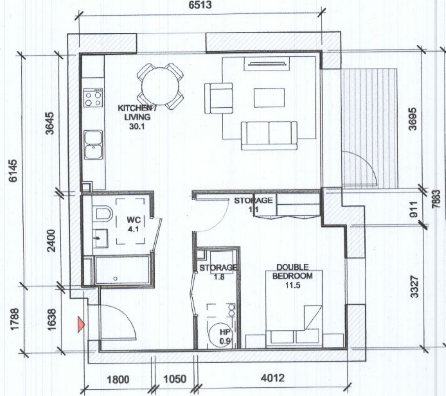
3 T.103 C 1:100
