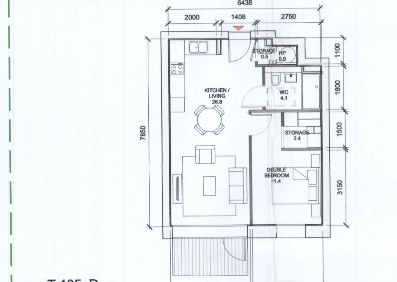
13 T.105 D 1:100
