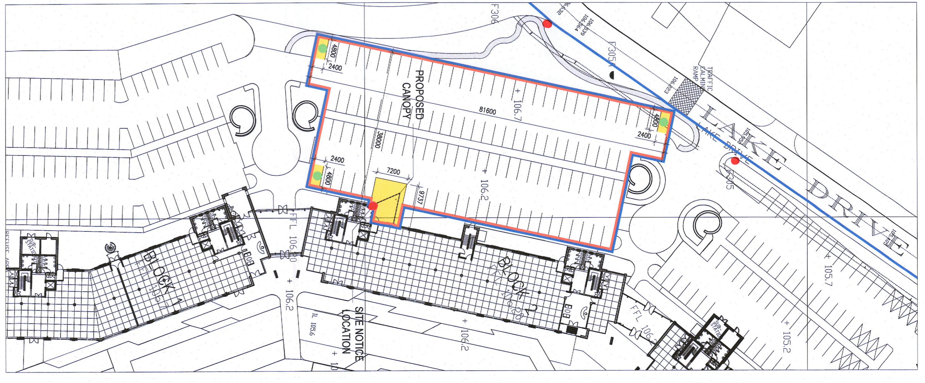
2 SITE LAYOUT PLAN Scale: 1:500
