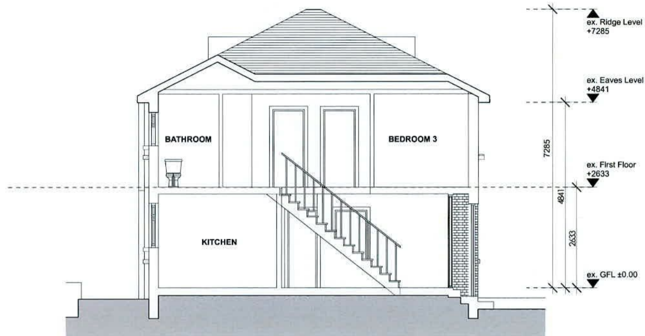
1 Existing Section A-A Scale: 1:100
