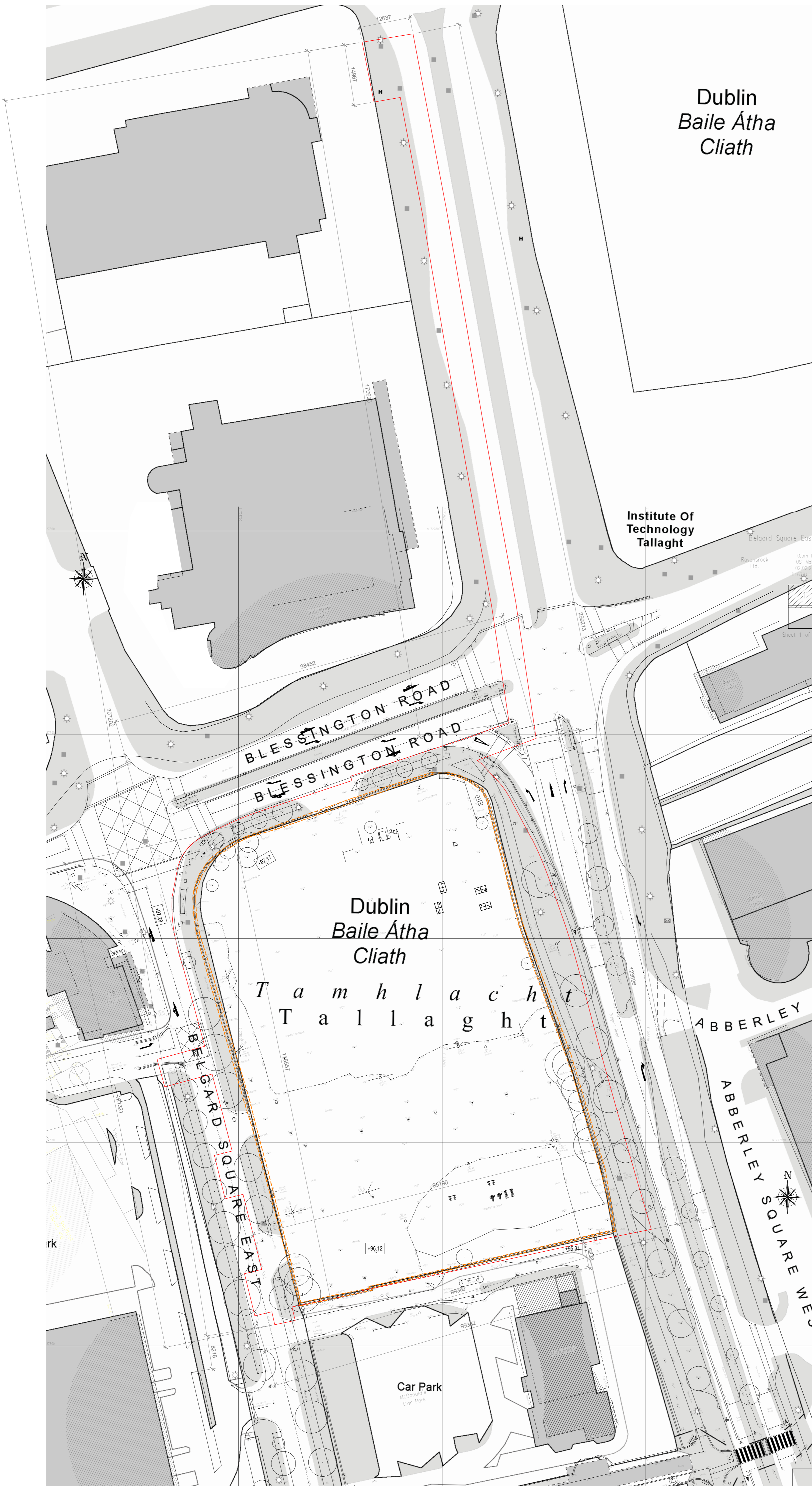
1 SITE - EXISTING SITE LAYOUT PLAN 1 : 500
