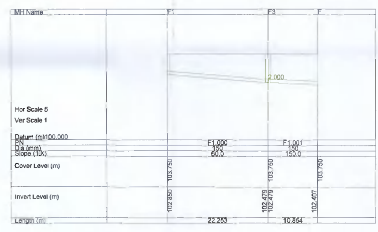
BASEMENT NETWORK: F1.000 - F1.002
