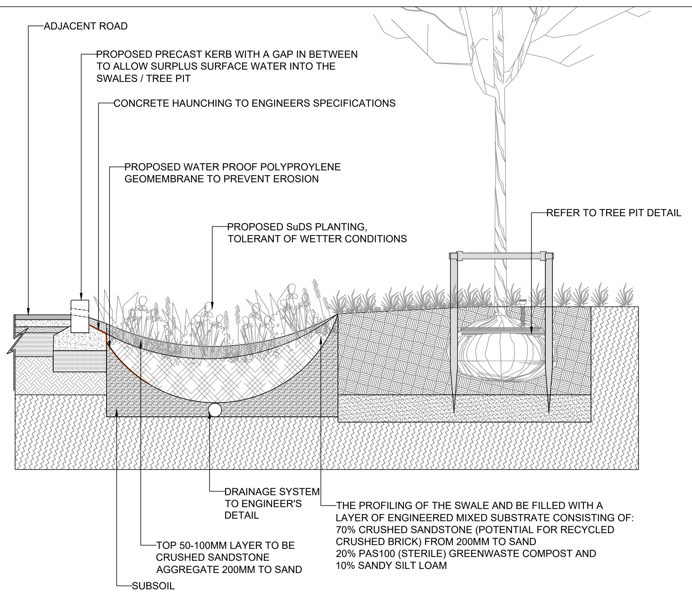
Section D-D scale 1:20 @A1
