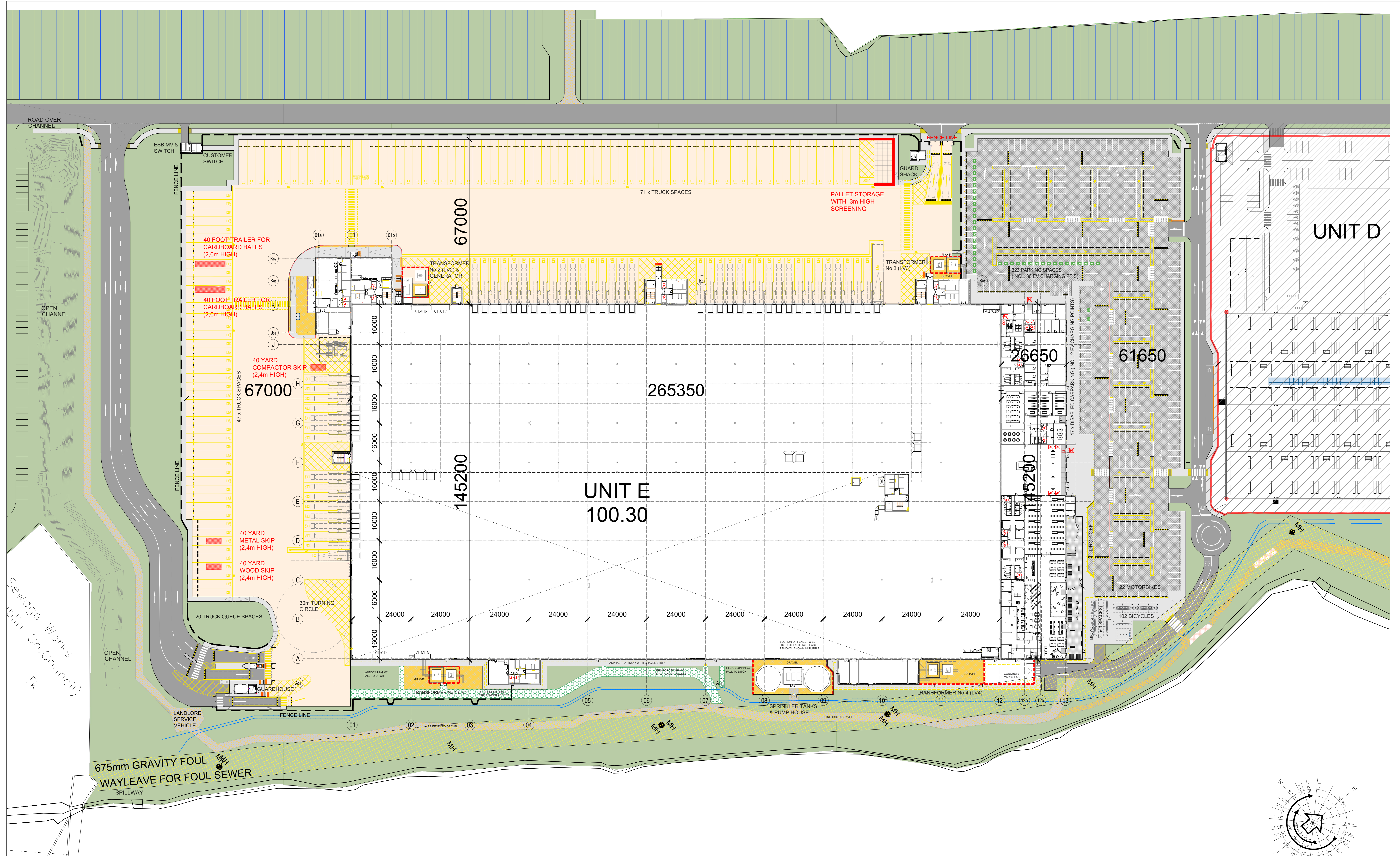
SITE PLAN 1:500
