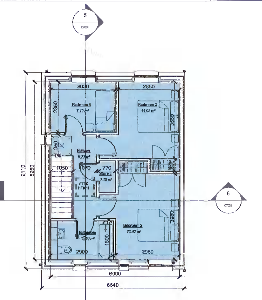
3 Level 02 Scale: 1:100
