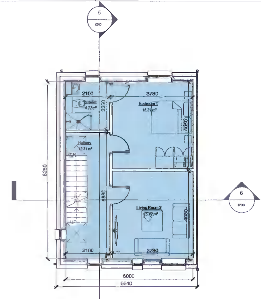
2 Level 01 Scale: 1:100
