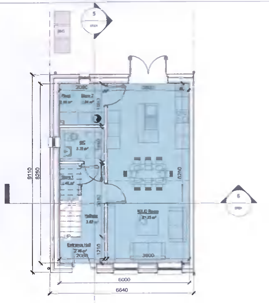
1 Level 00 Scale: 1:100
