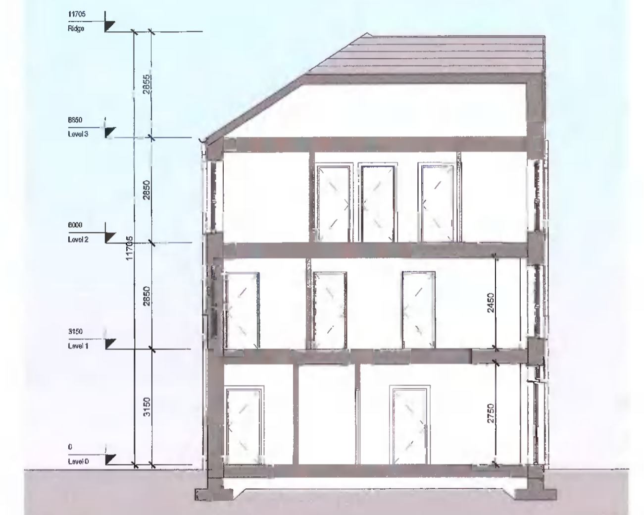
5 Section A-A Scale: 1:100
