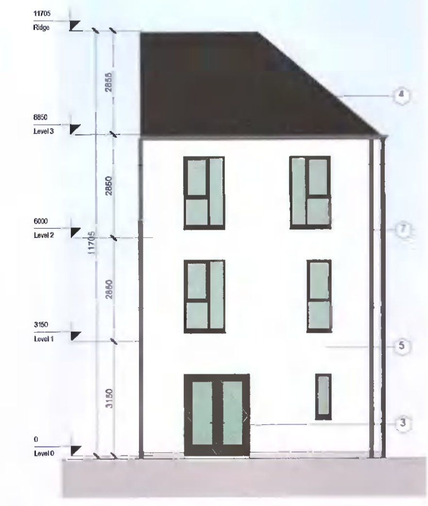
9 Rear Elevation Scale: 1:100
