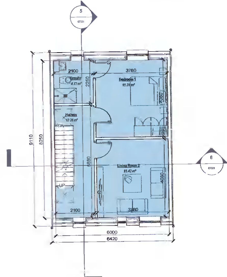
2 Level 01 Scale: 1:100
