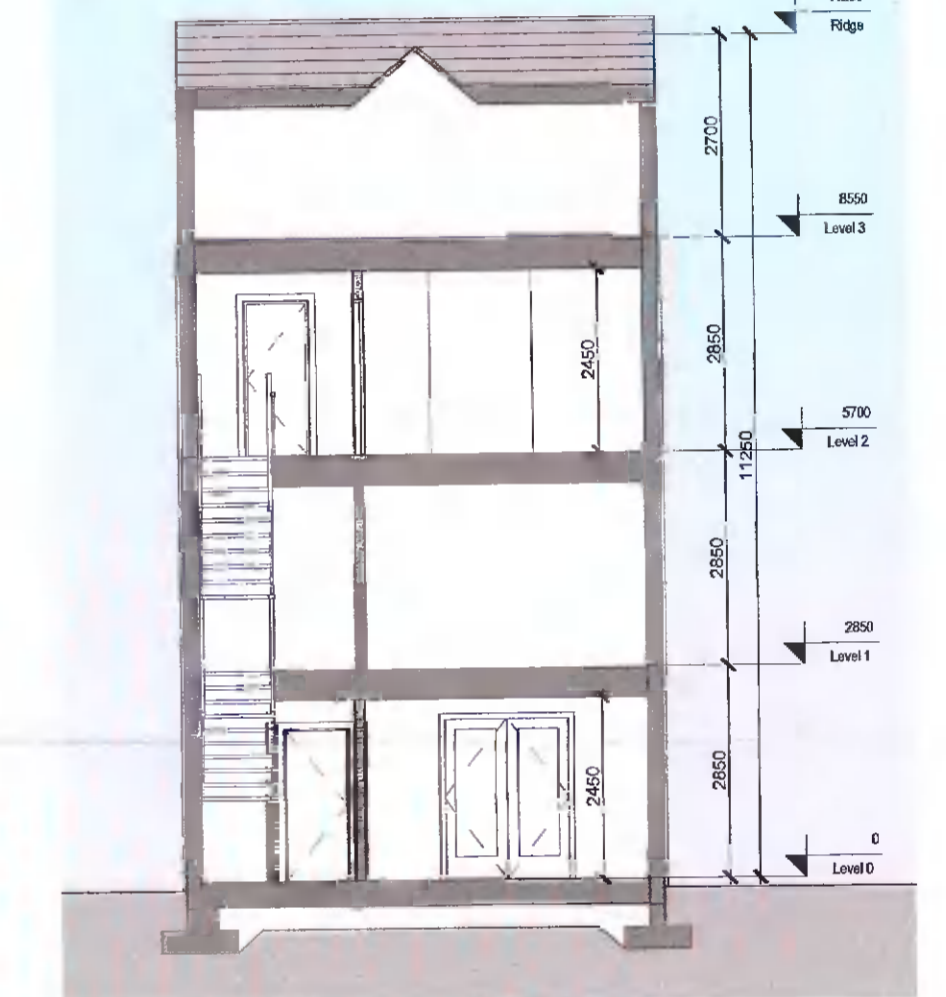
6 Section B-B Scale: 1:100
