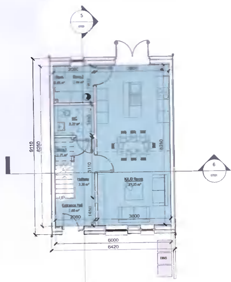
1 Level 00 Scale: 1:100
