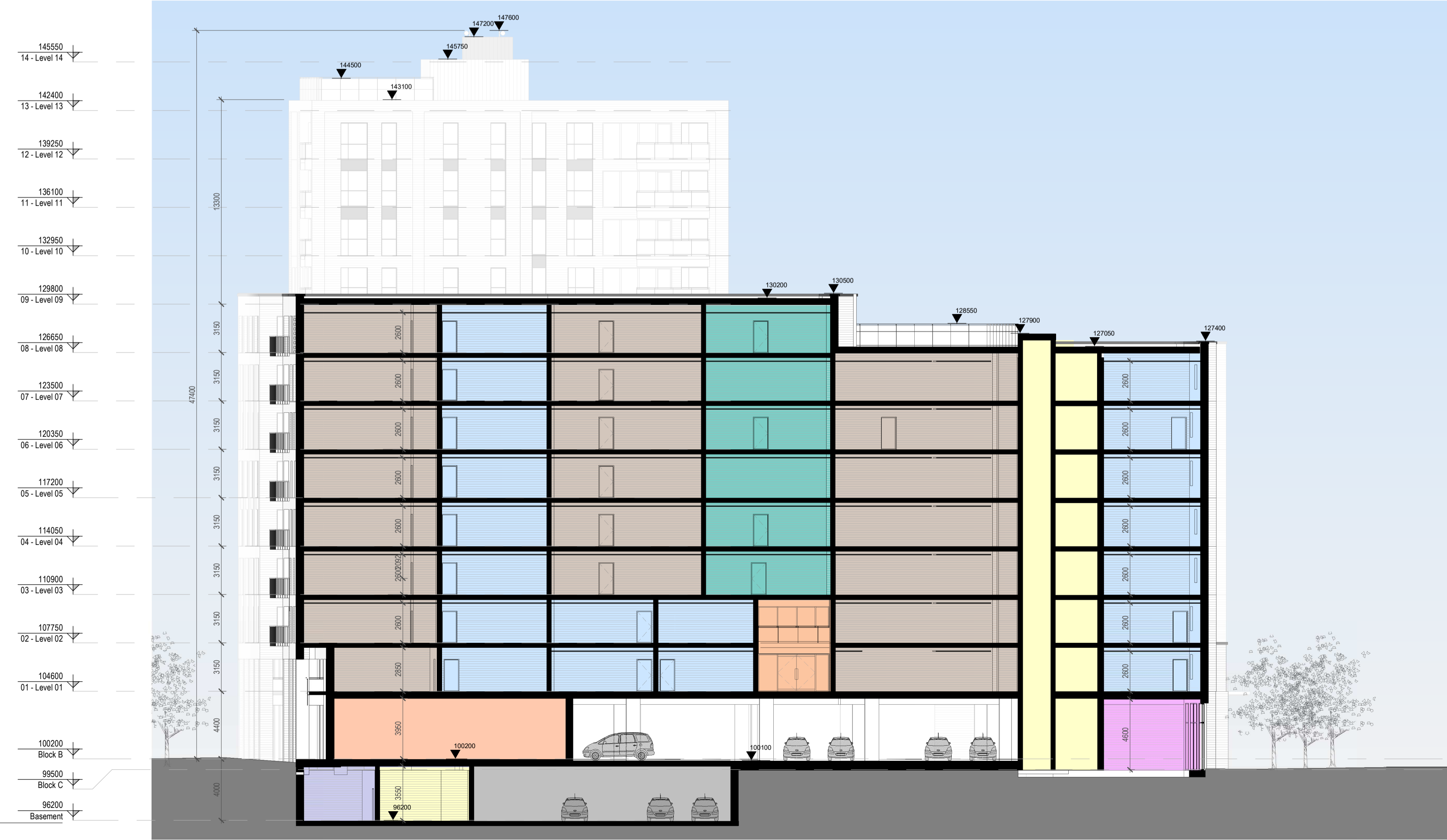
2 Section 02 1 : 200
