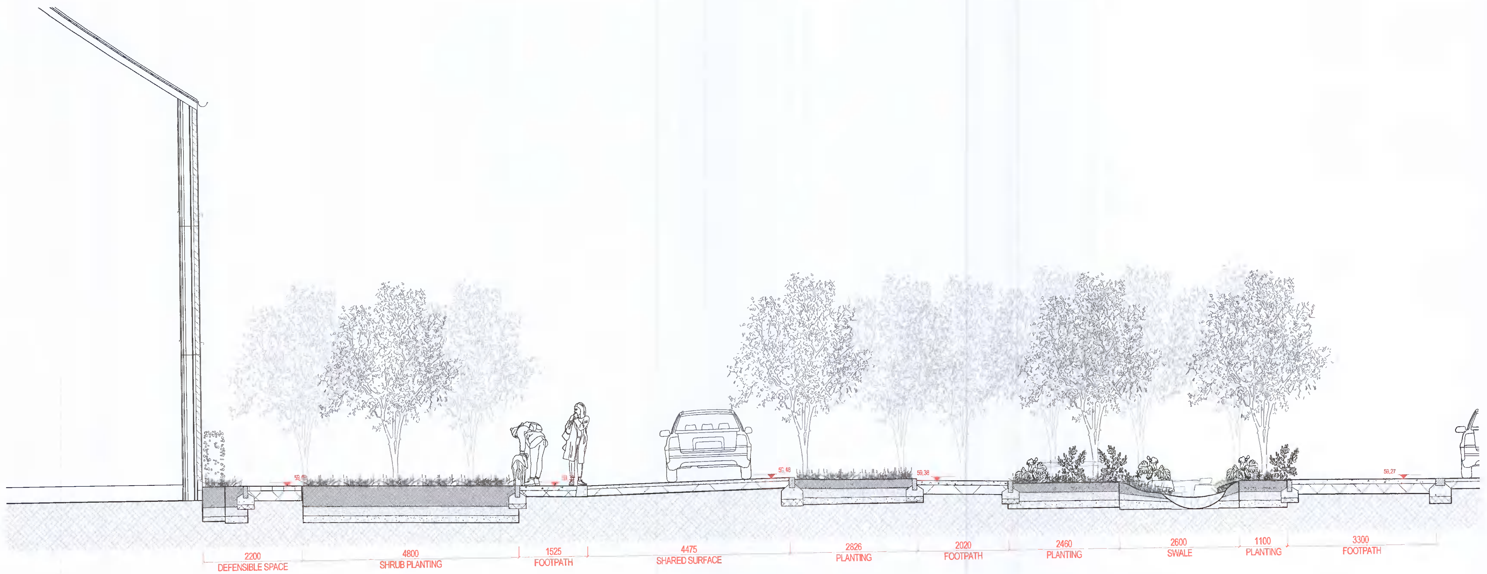
11 Section 11 1:50 @A1
