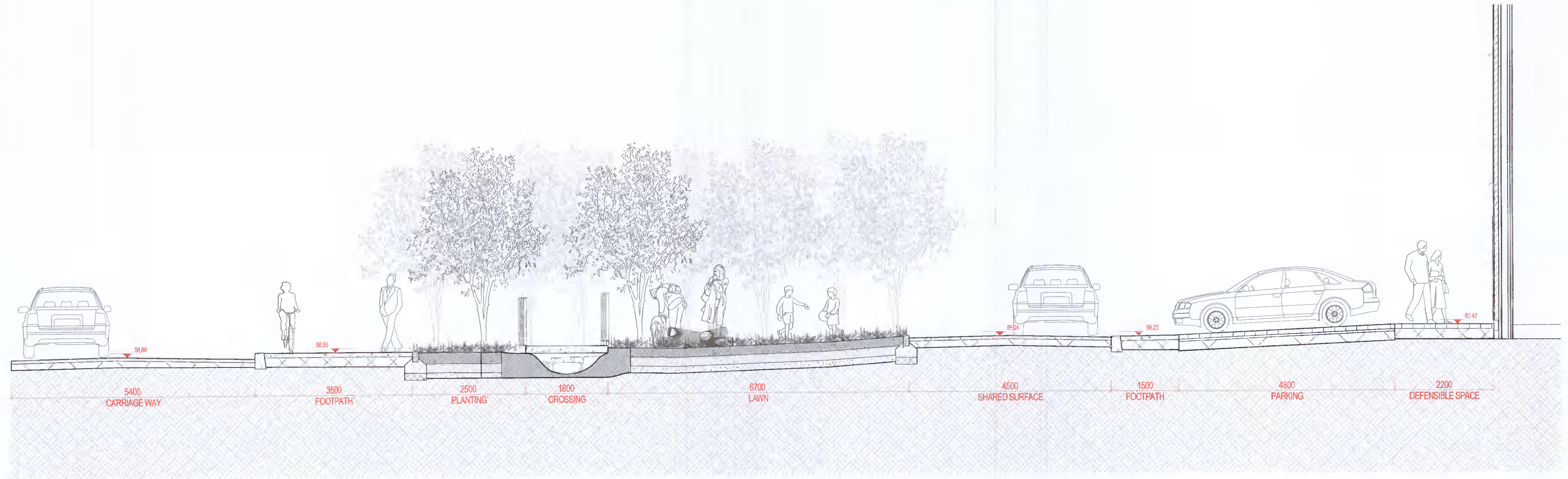
10 Section 10 1:50 @A1
