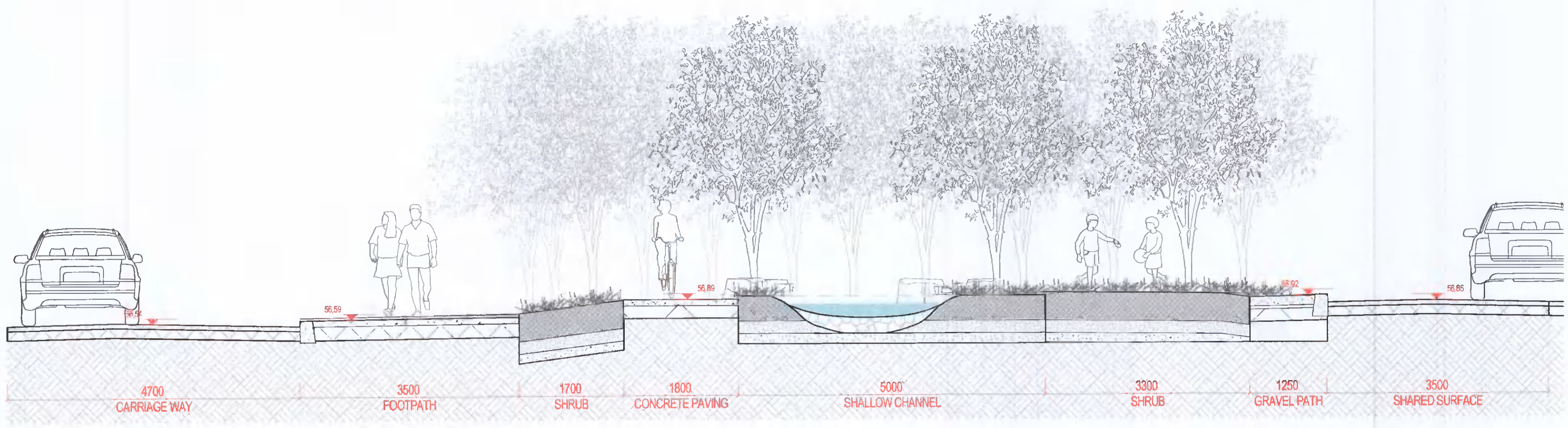
09 Section 09 1:50 @A1
