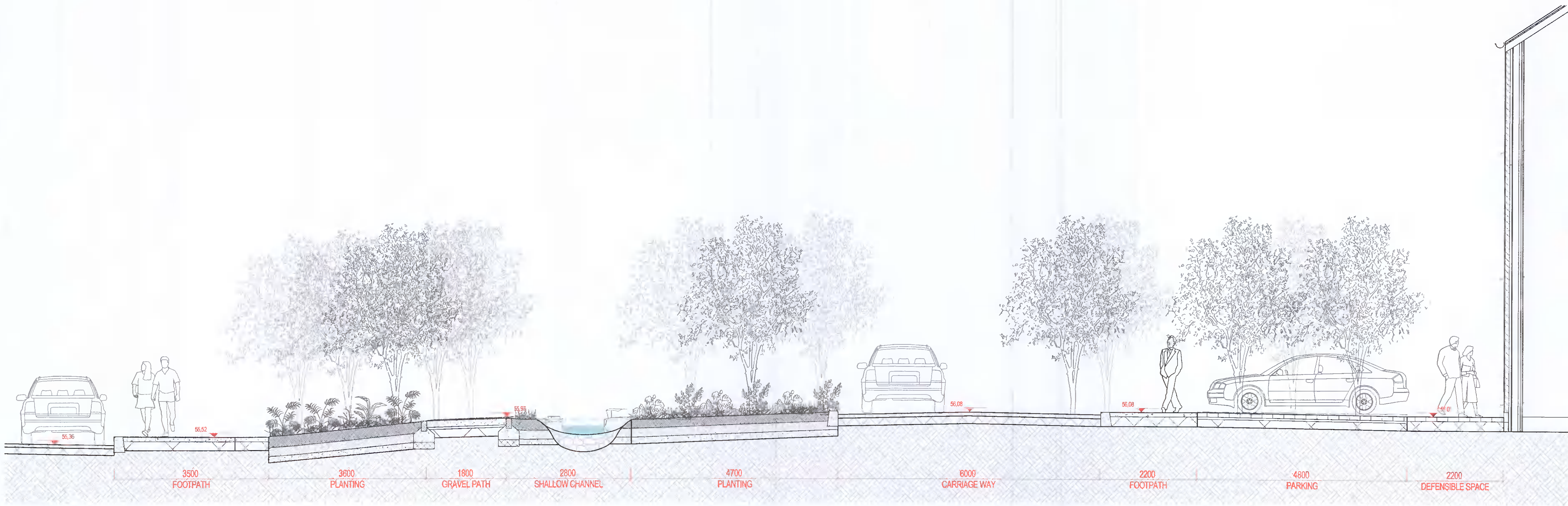
08 Section 08 1:50 @A1
