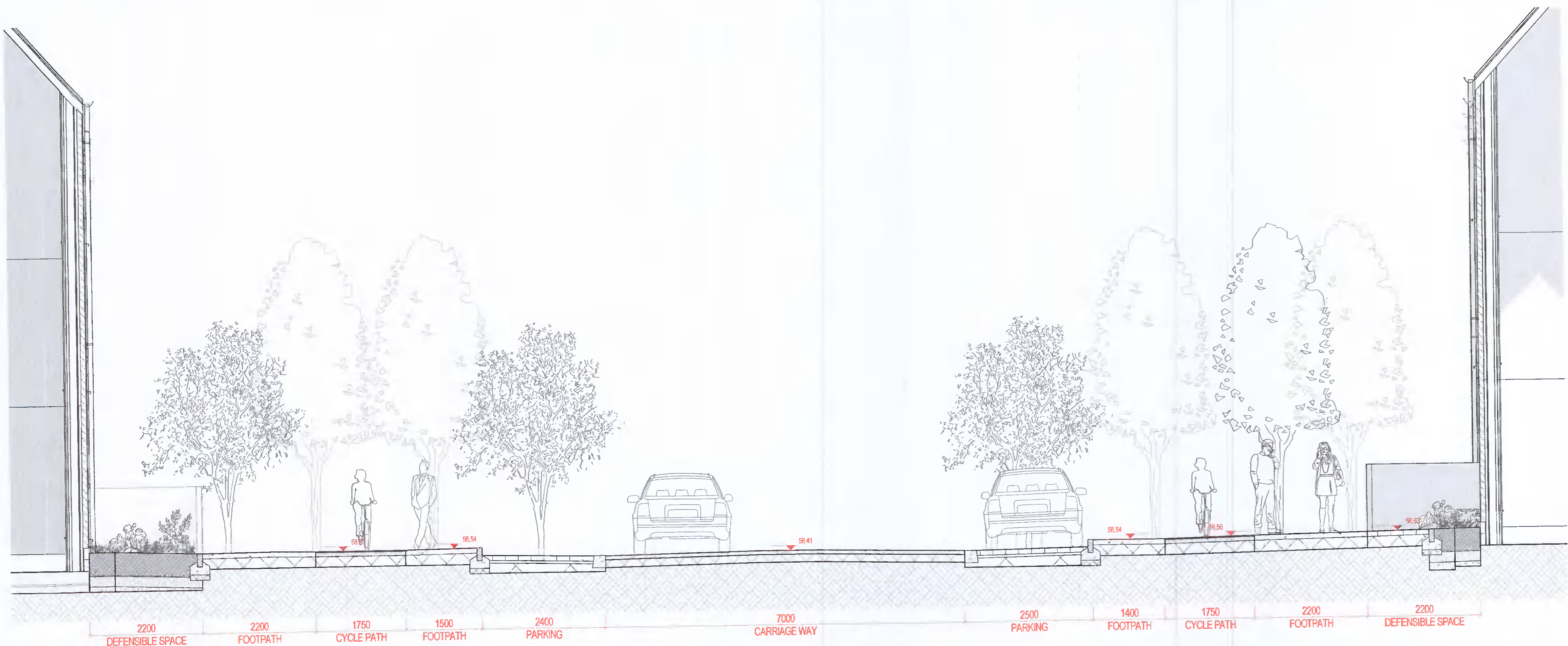
04 Section 04 1:50 @A1
