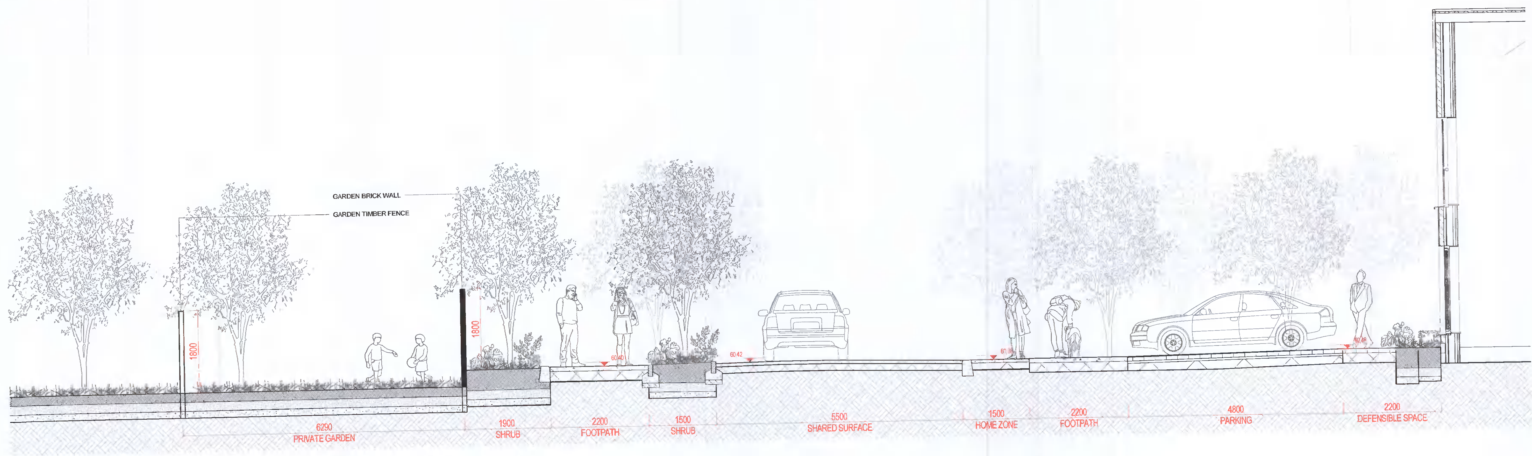
02 Section 02 1:50 @A1
