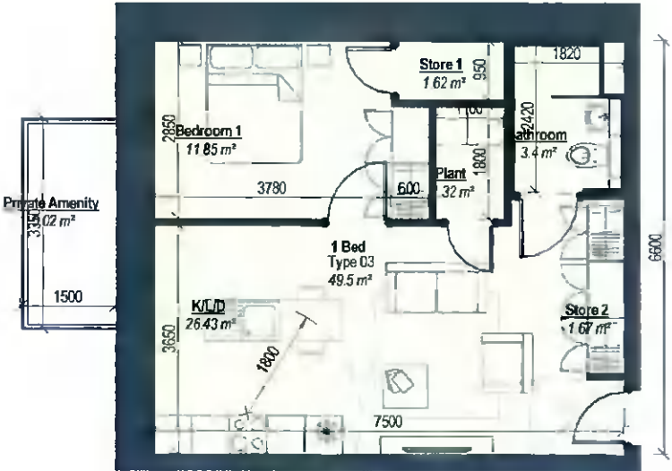
1 1 Bed Apt Type 03 Scale: 1 : 100
