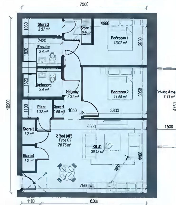
1 2 Bed Apt Type 01 Scale: 1 : 100
