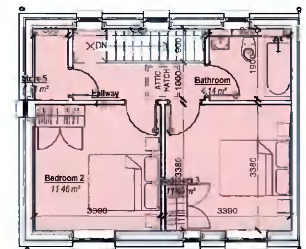
3 H3D - Level 02 Scale: 1 : 100
