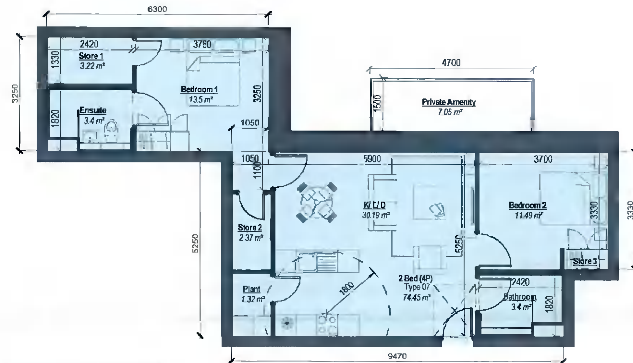
1 2 Bed Apt Type 07 Scale: 1 : 100
