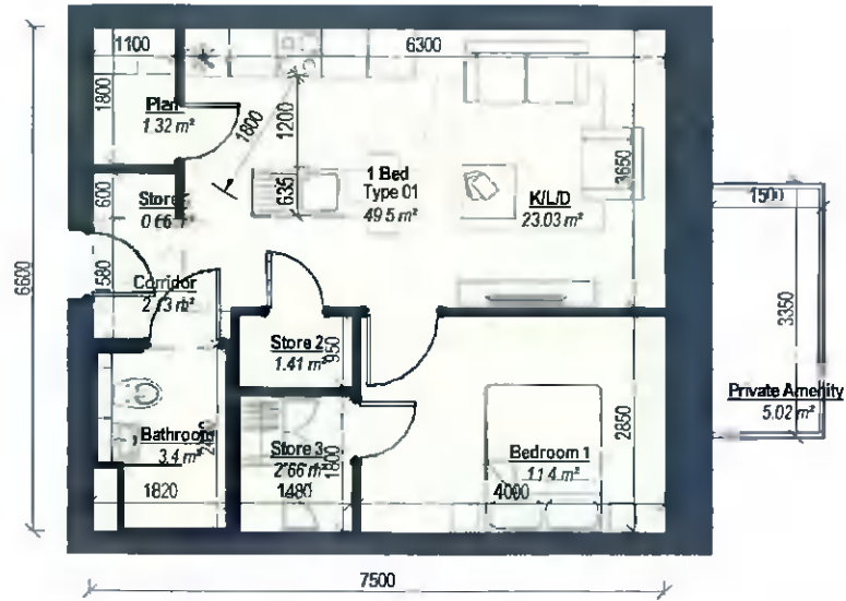
1 1 Bed Apt Type 01 Scale: 1 : 100
