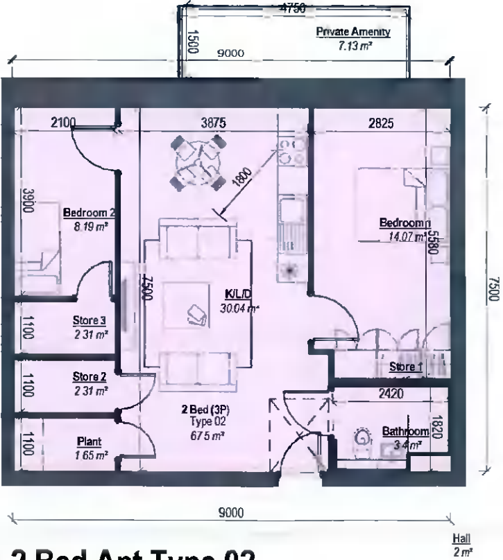
1 2 Bed Apt Type 02 Scale: 1 : 100
