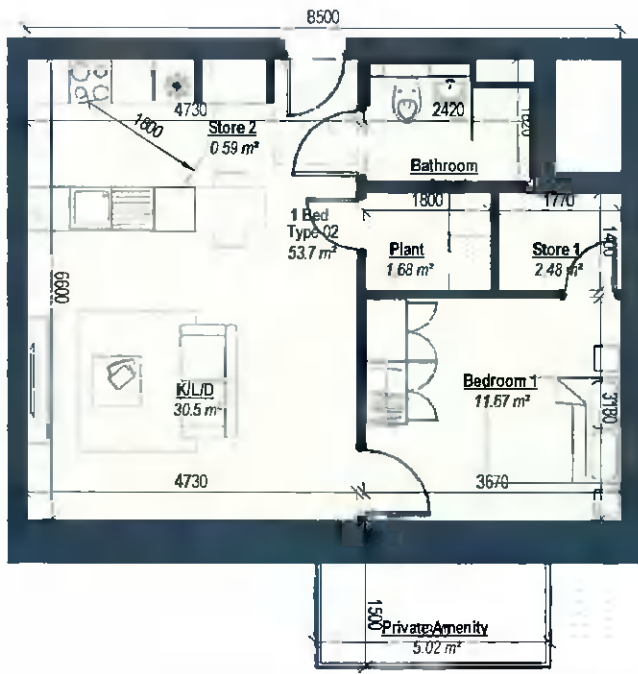
1 1 Bed Apt Type 02 Scale: 1 : 100
