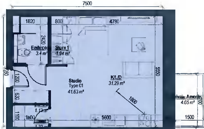
1 Studio Apt Type 01 Scale: 1 : 100
