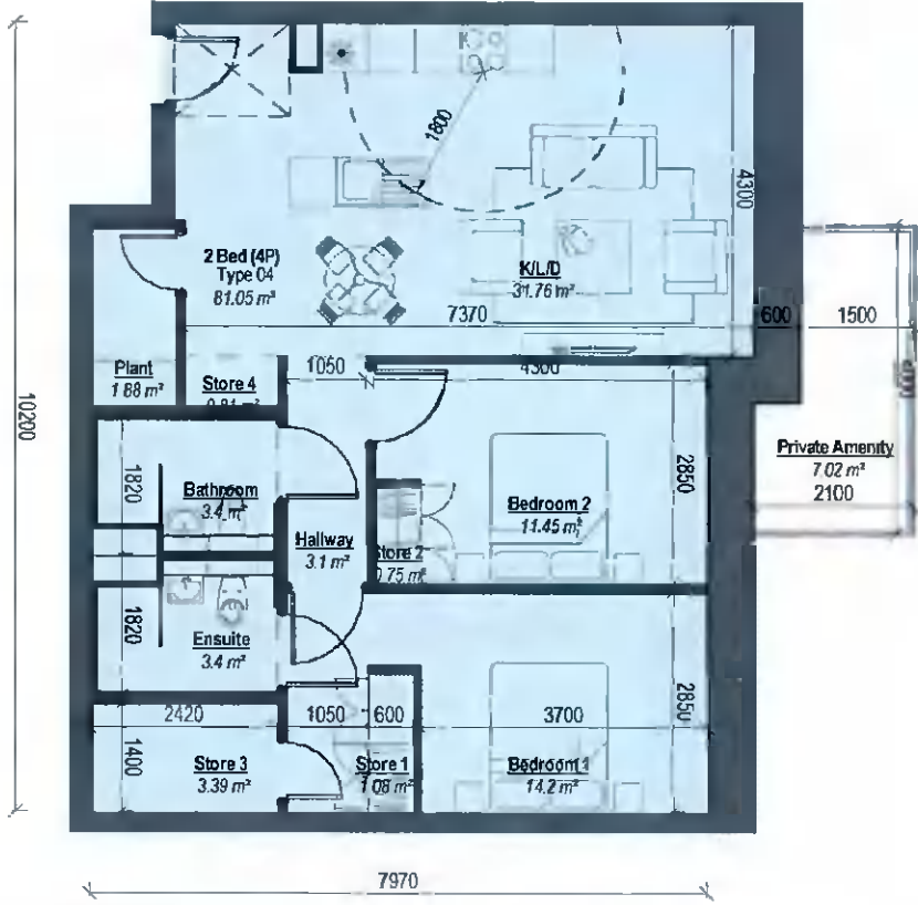
1 2 Bed Apt Type 04 Scale: 1 : 100
