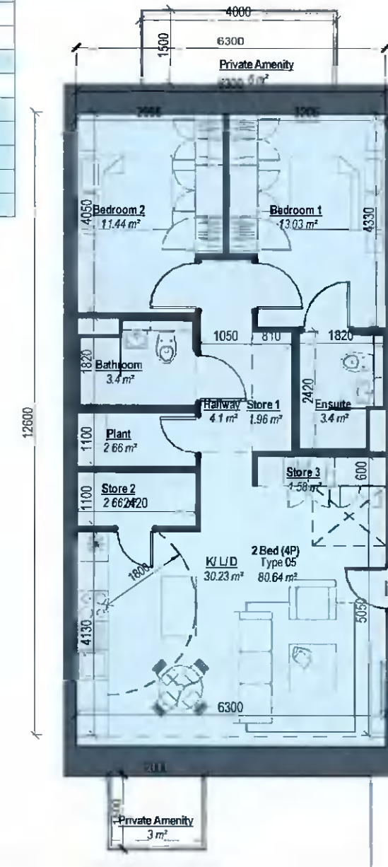
1 2 Bed Apt Type 05 Scale: 1:100
