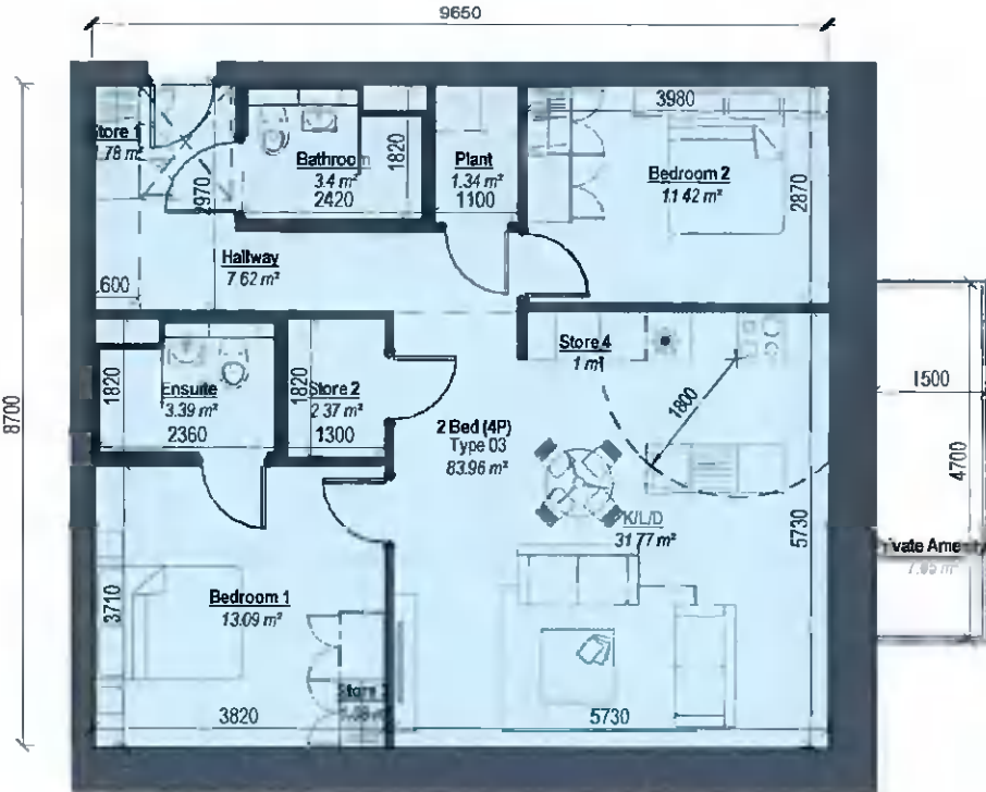
1 2 Bed Apt Type 03 Scale: 1 : 100
