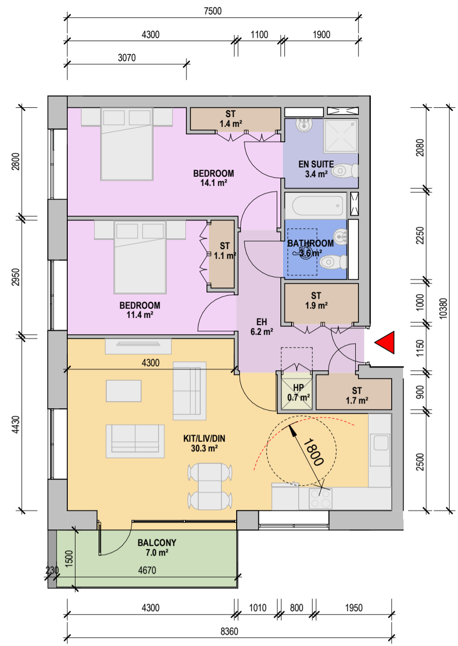
1 APT TYPE - 2A 1 : 100
