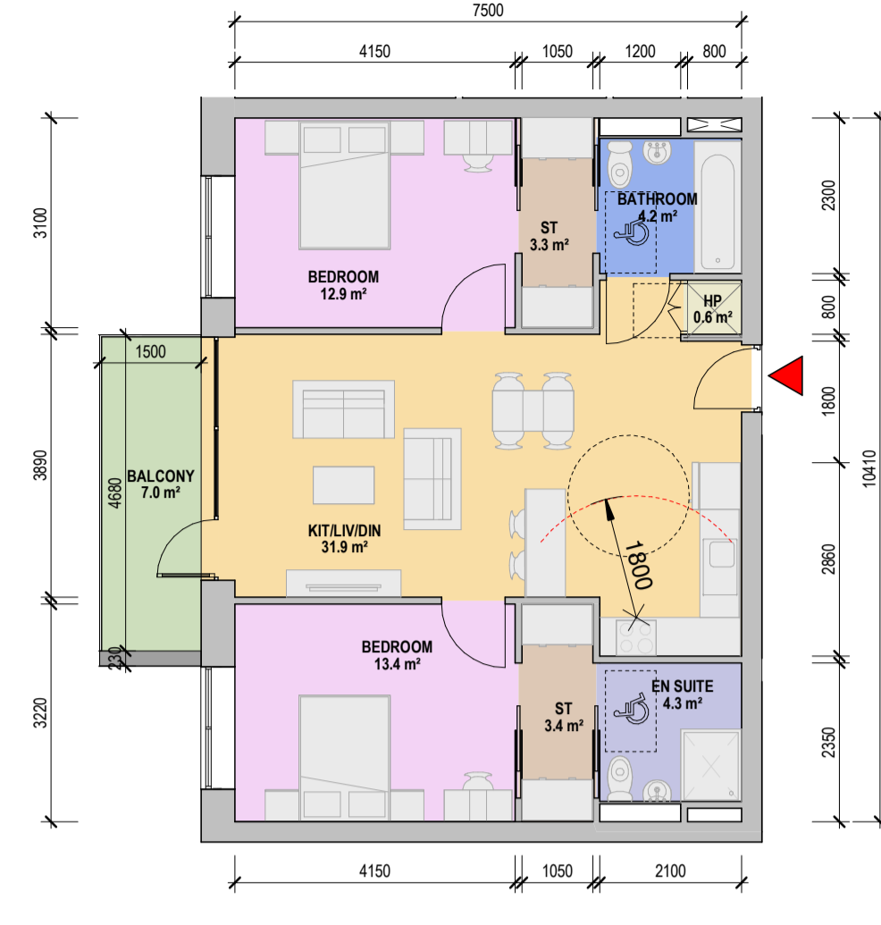
3 APT TYPE - 2C 1 : 100
