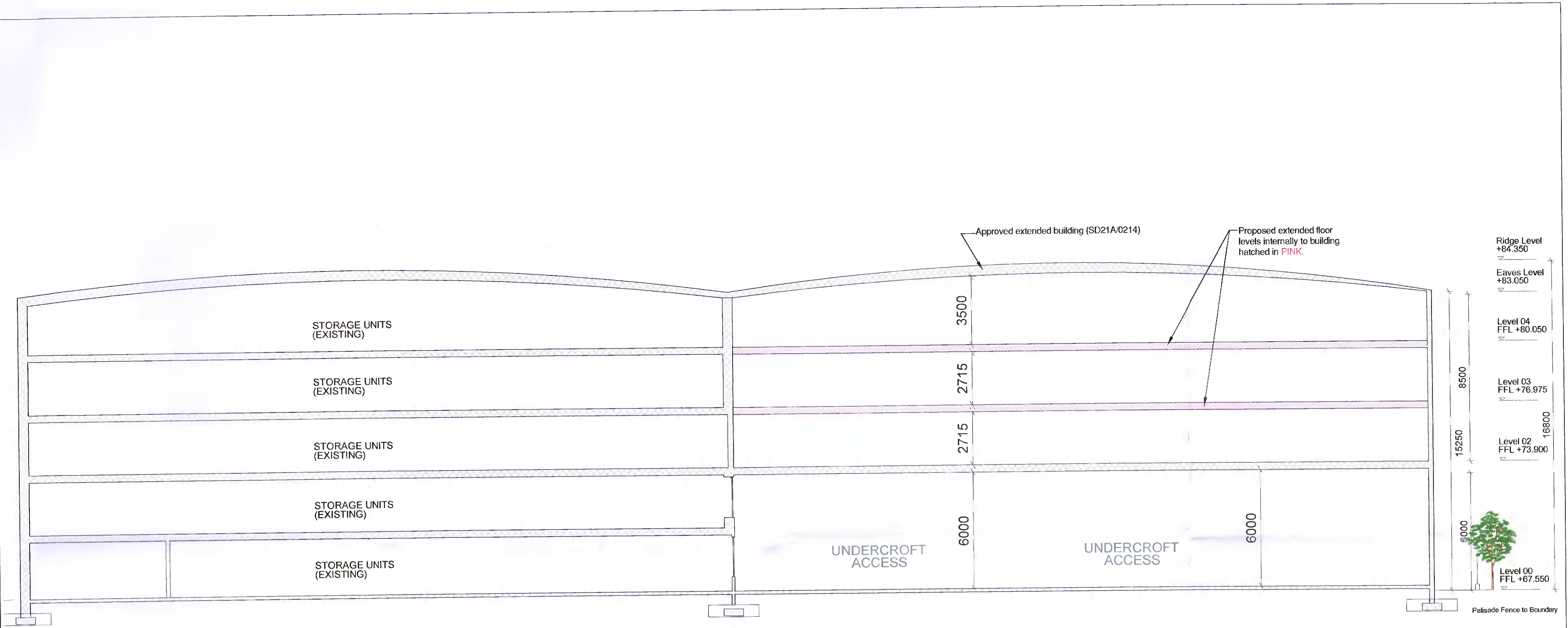
01 Section A-A A-A 1:100
