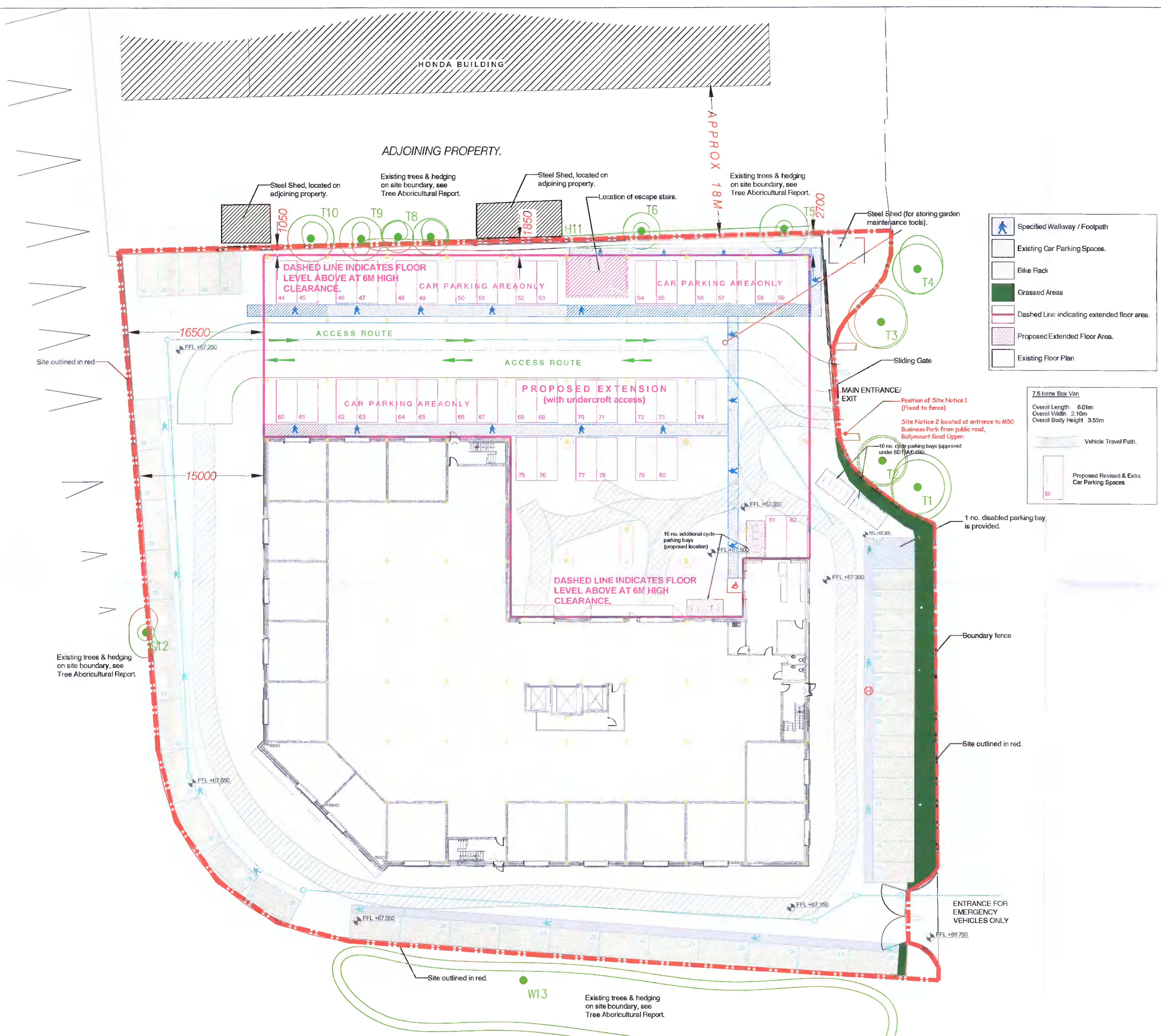
Site Layout Plan (Scale 1:250).
