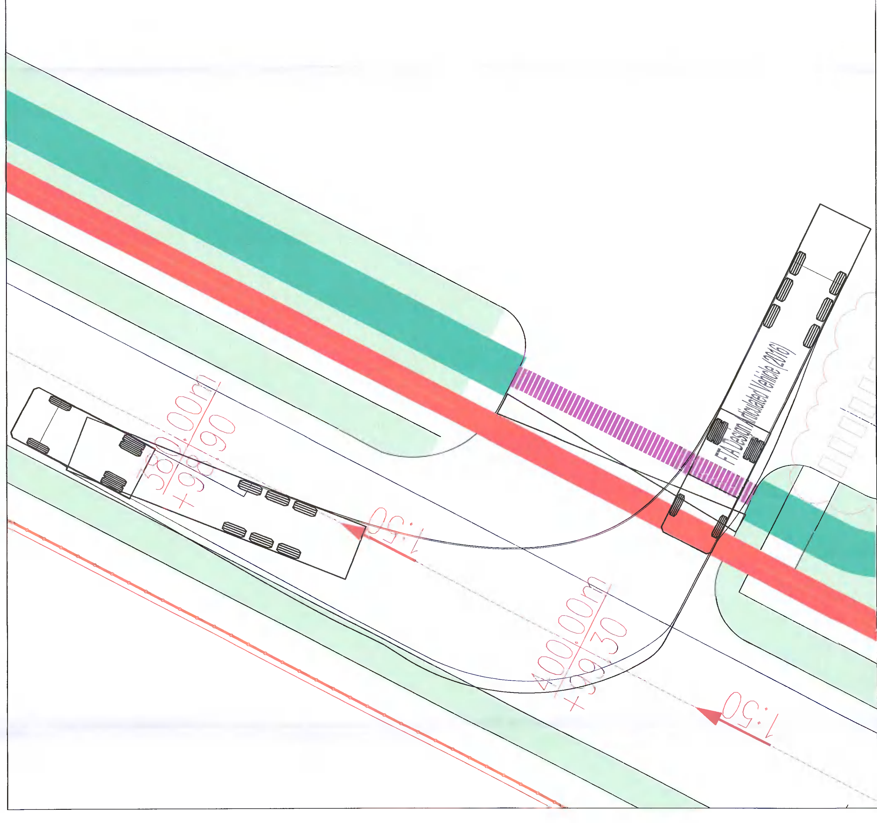
HGV SITE B2 EGRESS - SCALE 1:100
