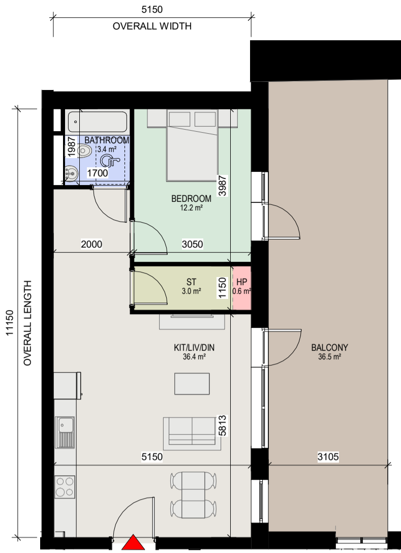
3 Apartment Type 1R 1 : 100
