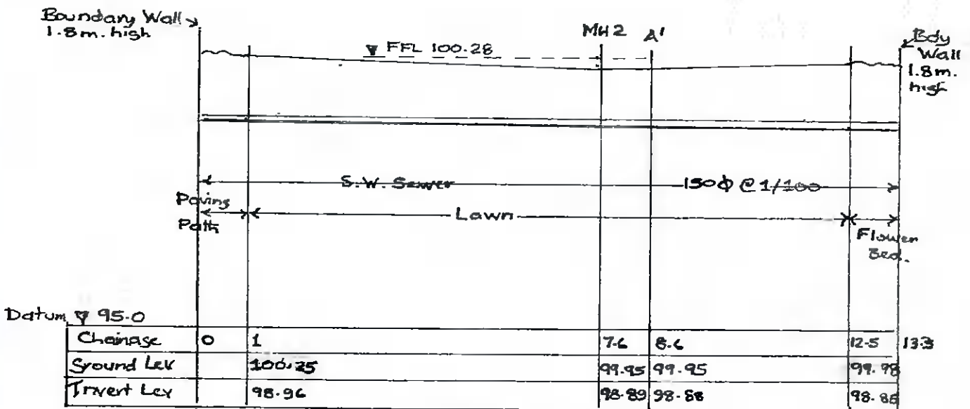
Scales Hor 1/100 Ver 1/100 Longitudinal Section 150 \phi S.W. Sewer
