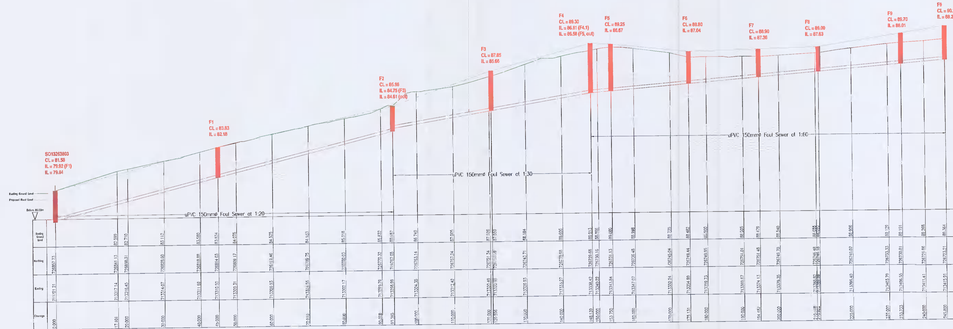
FOUL SEWER F1 TO F9 LONGITUDINAL SECTION Scale 1:500 Horizontal, 1:100 Vertical
