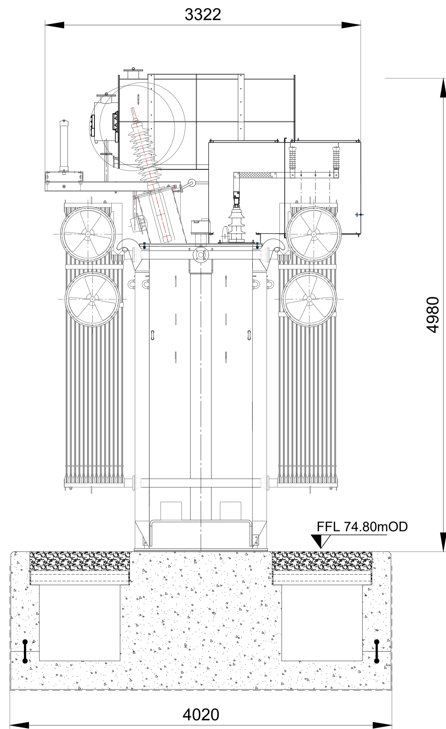
ELEVATION
