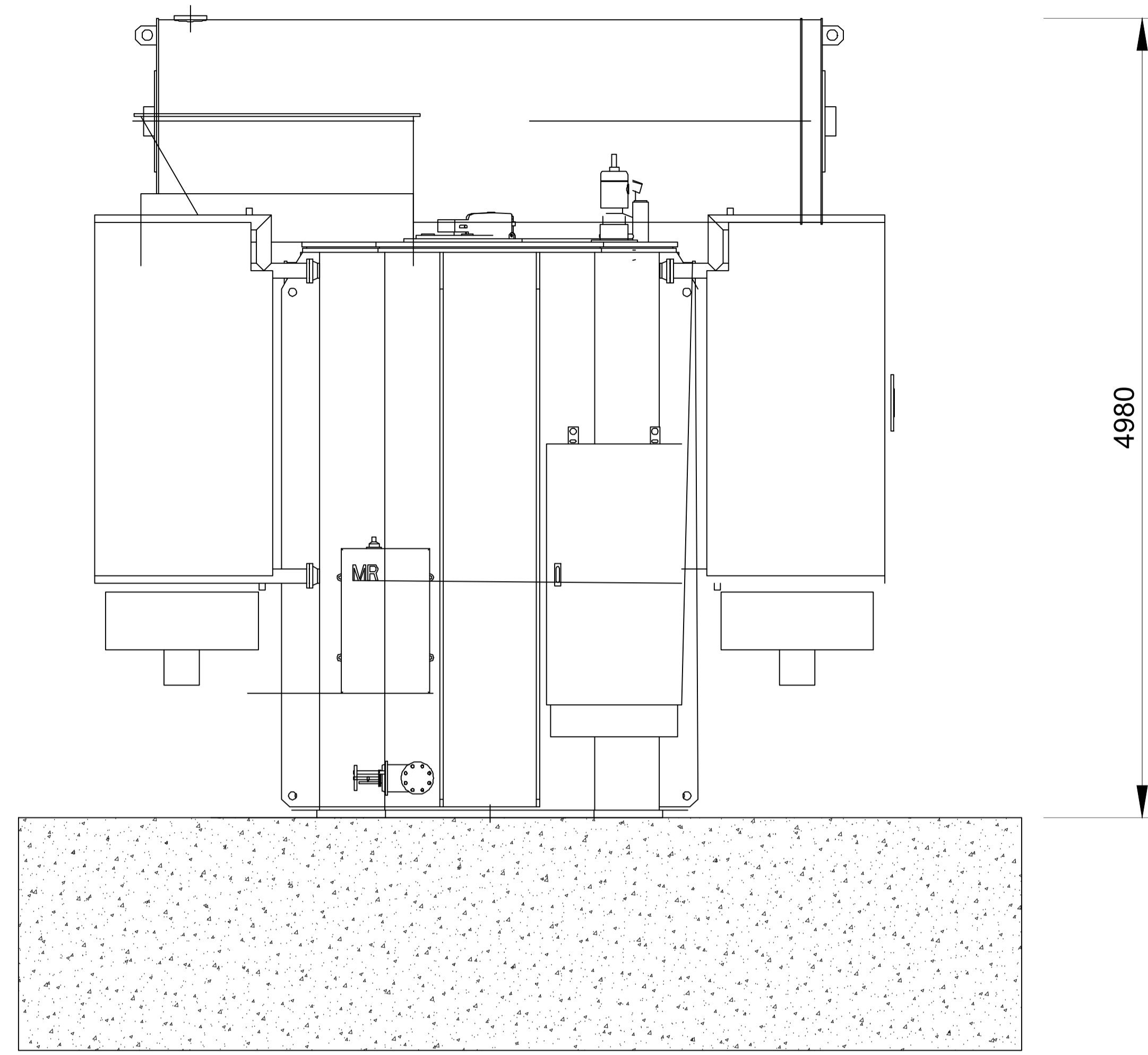
ELEVATION
