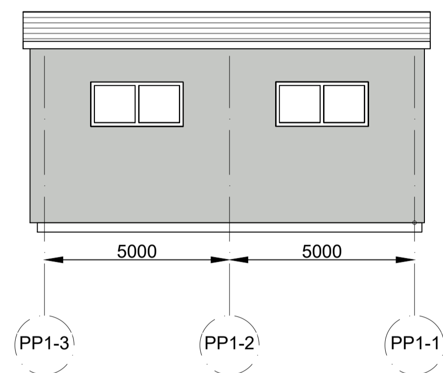
Elevation S4
