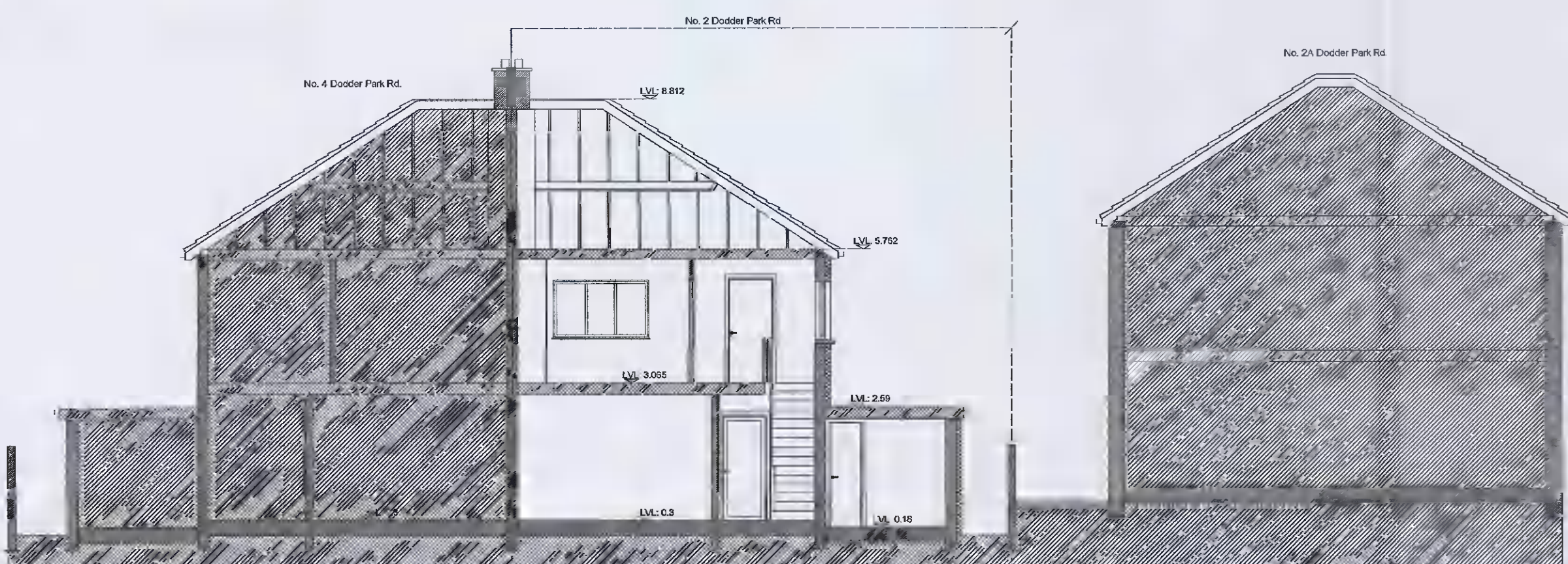
Section D-D
