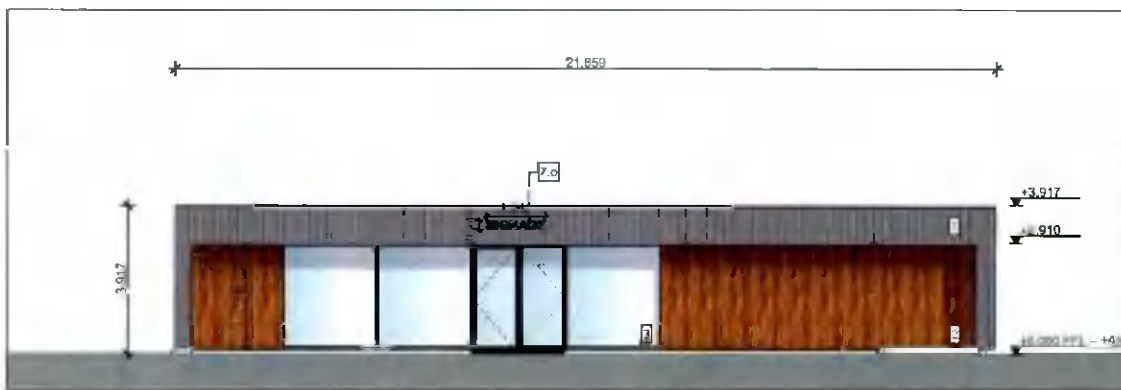
④ Elevation A 1:200
