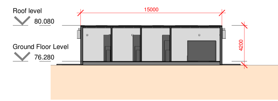
8 1007 Section BB 1 : 200
