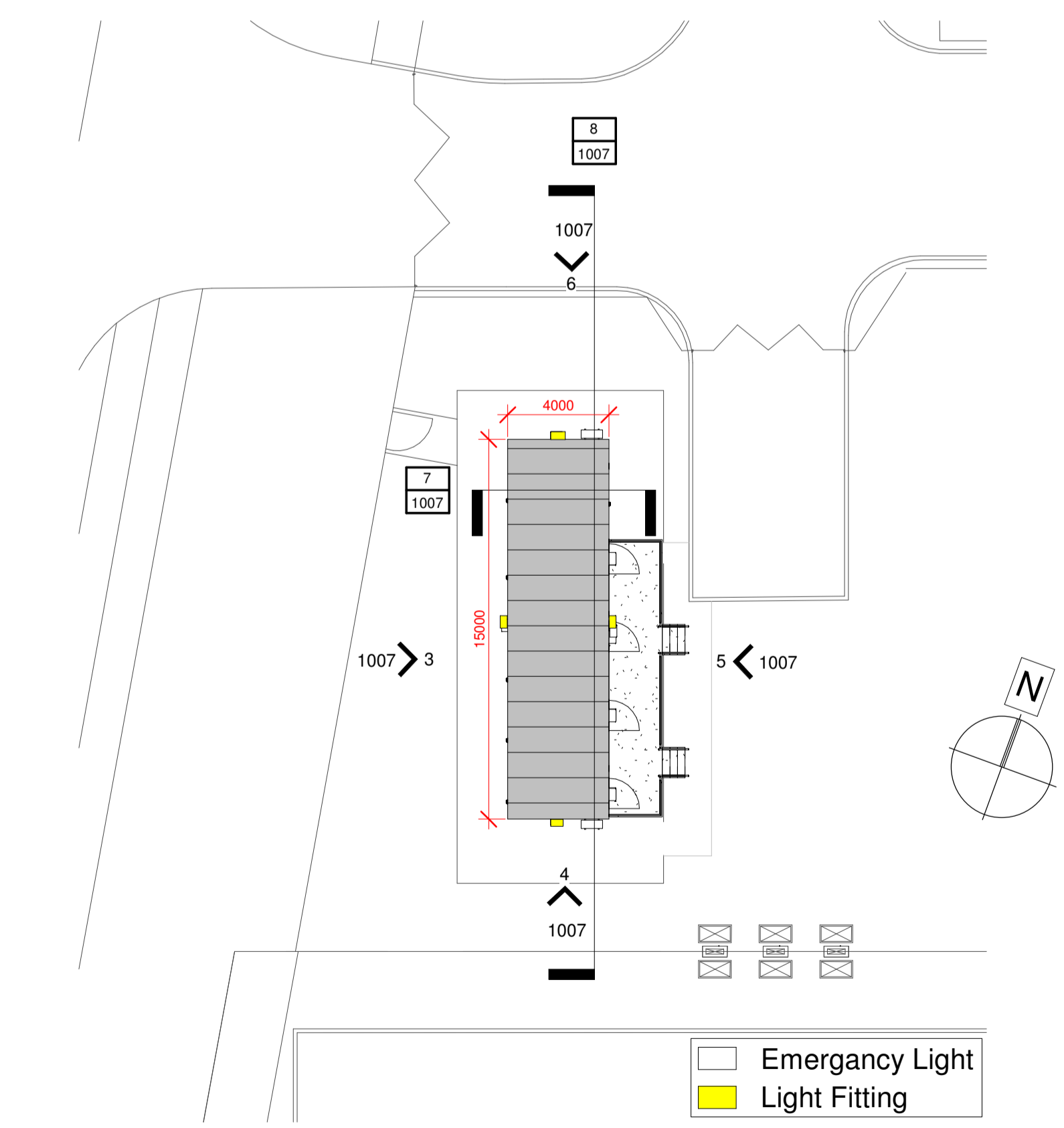
2 1007 Roof level 1 : 200
