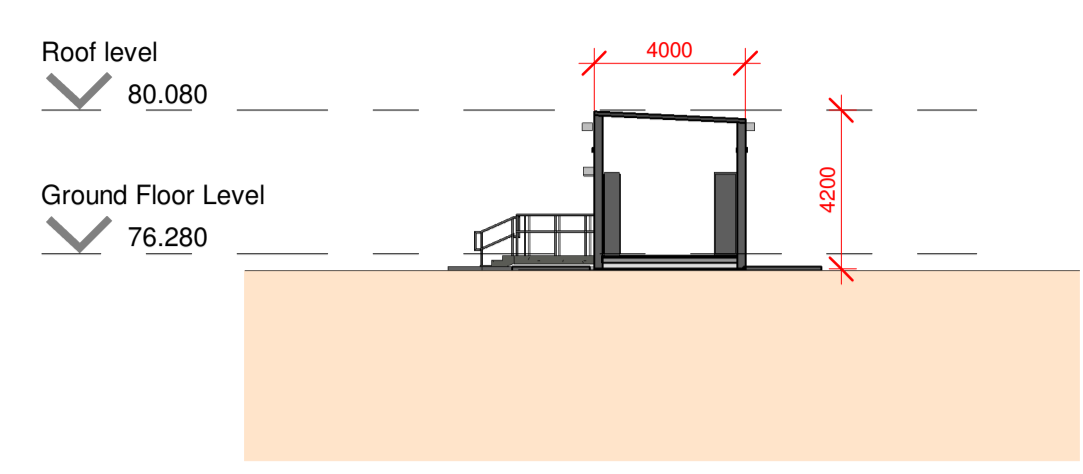
7 1007 Section AA 1 : 200
